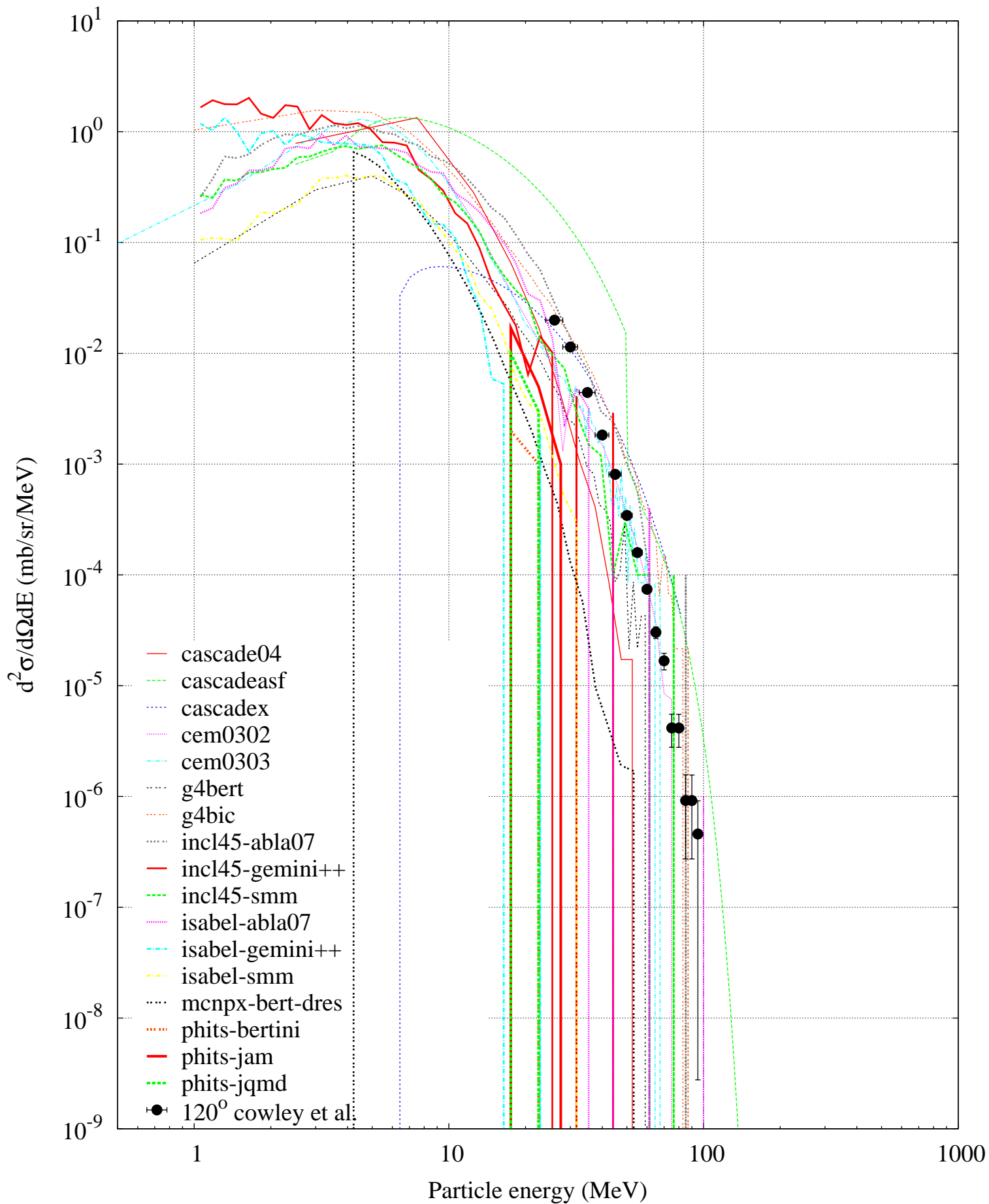
p (160 MeV) + Al -- Alpha spectrum
