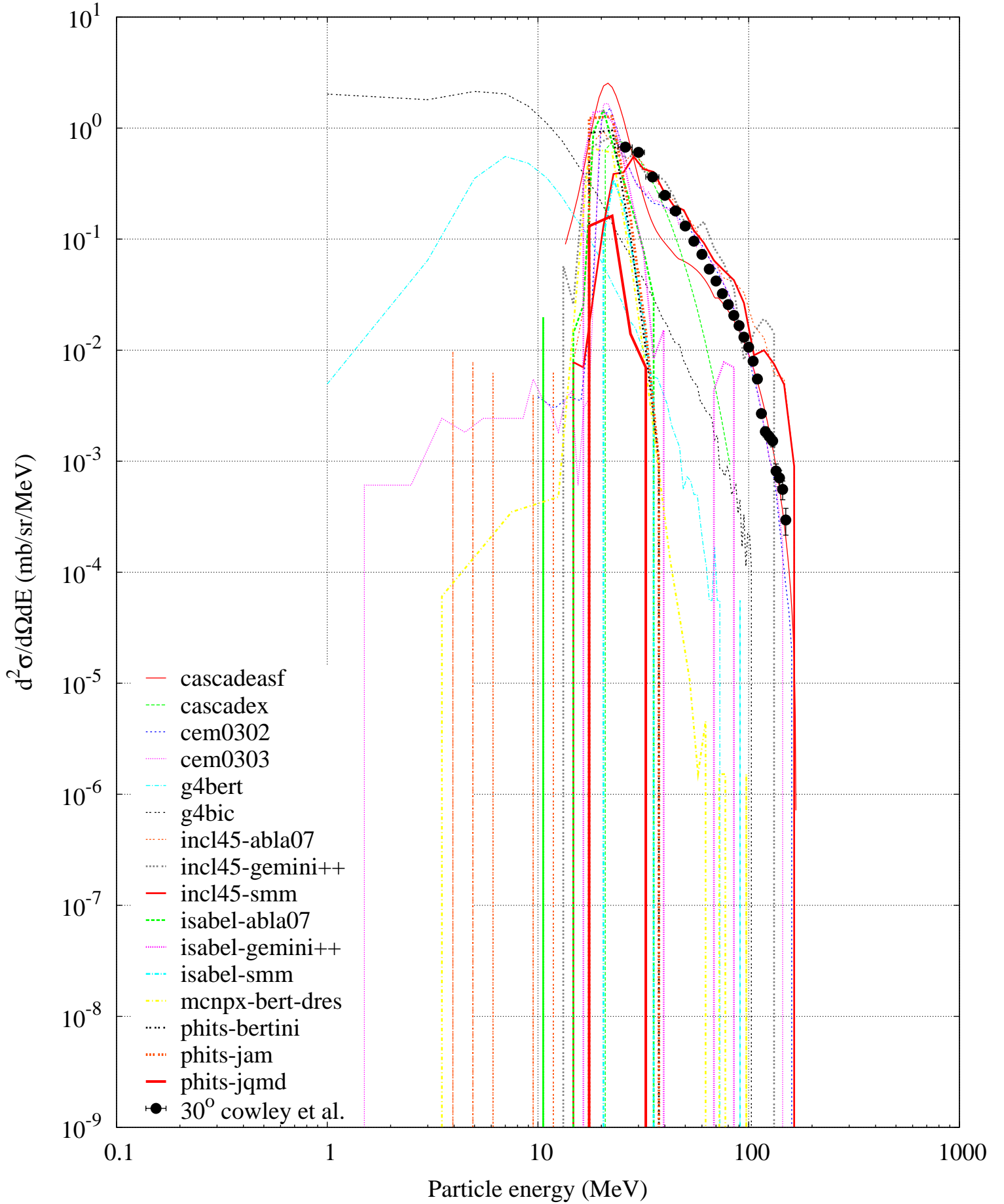
p (160 MeV) + Au -- Alpha spectrum
