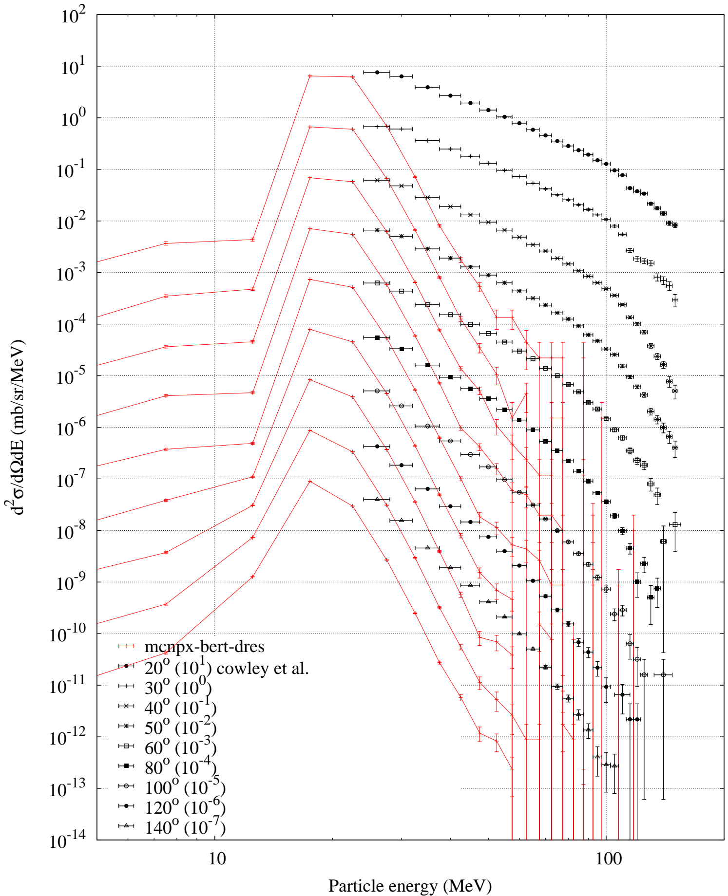
p (160 MeV) + Au -- Alpha spectrum
