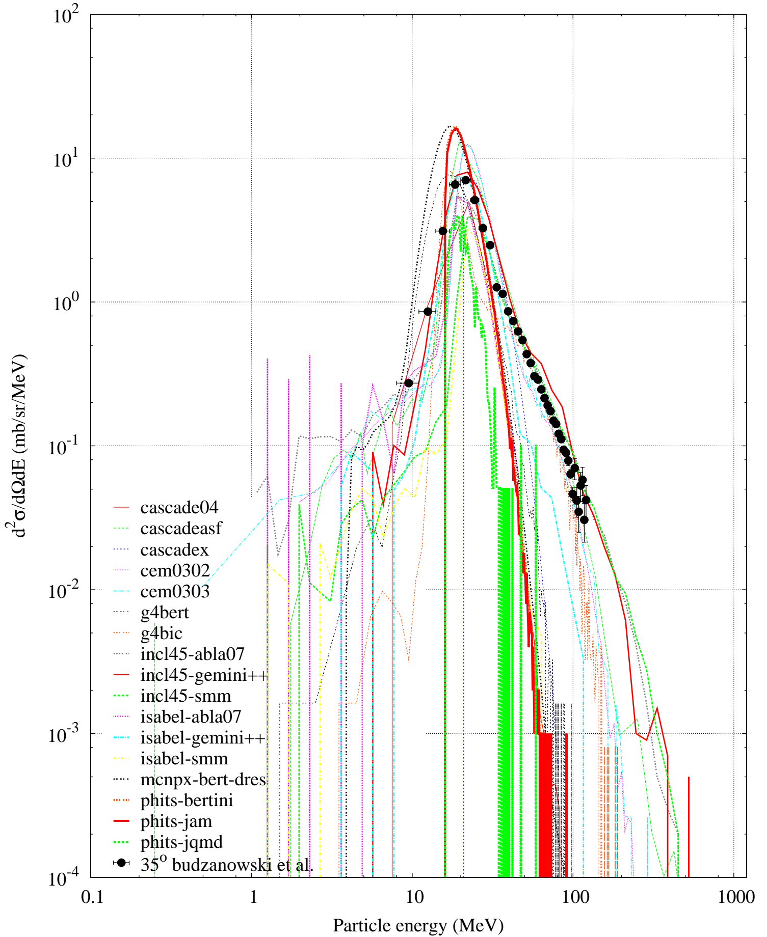
p (1200 MeV) + Au -- Alpha spectrum
