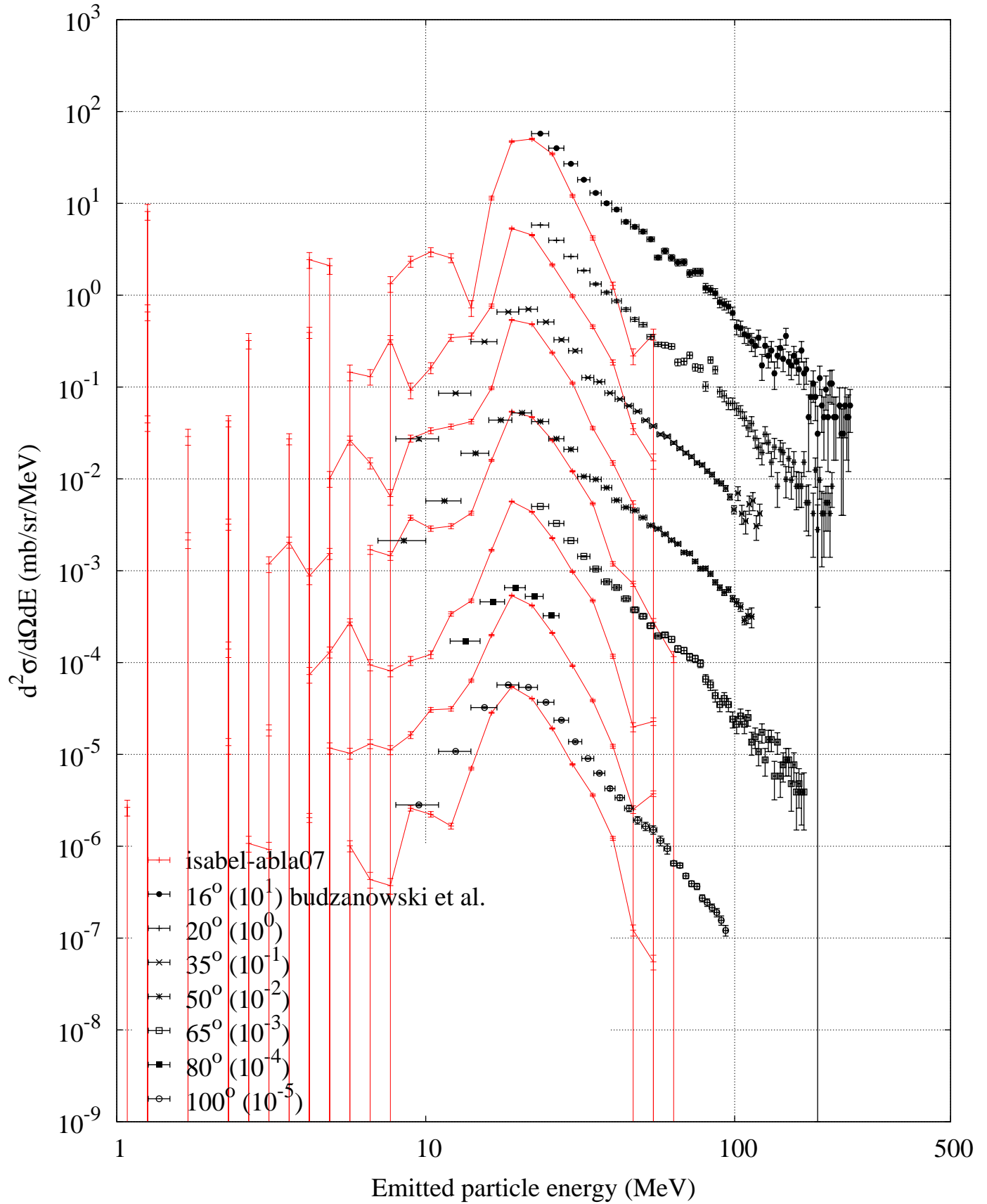
p (1200 MeV) + Au -- Helium-4 spectrum
