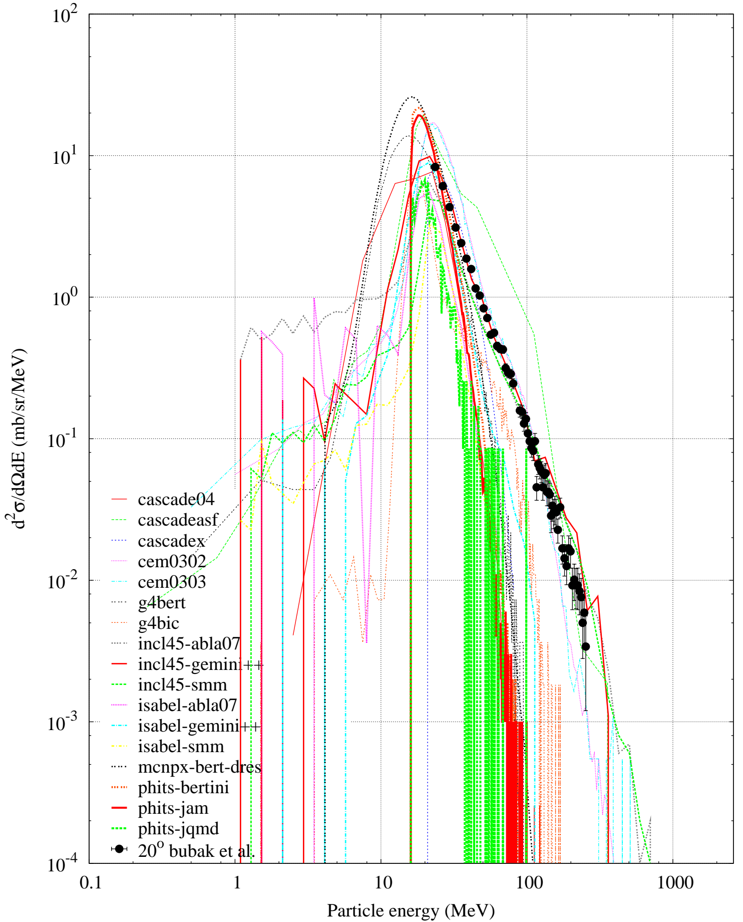
p (2500 MeV) + Au -- Alpha spectrum
