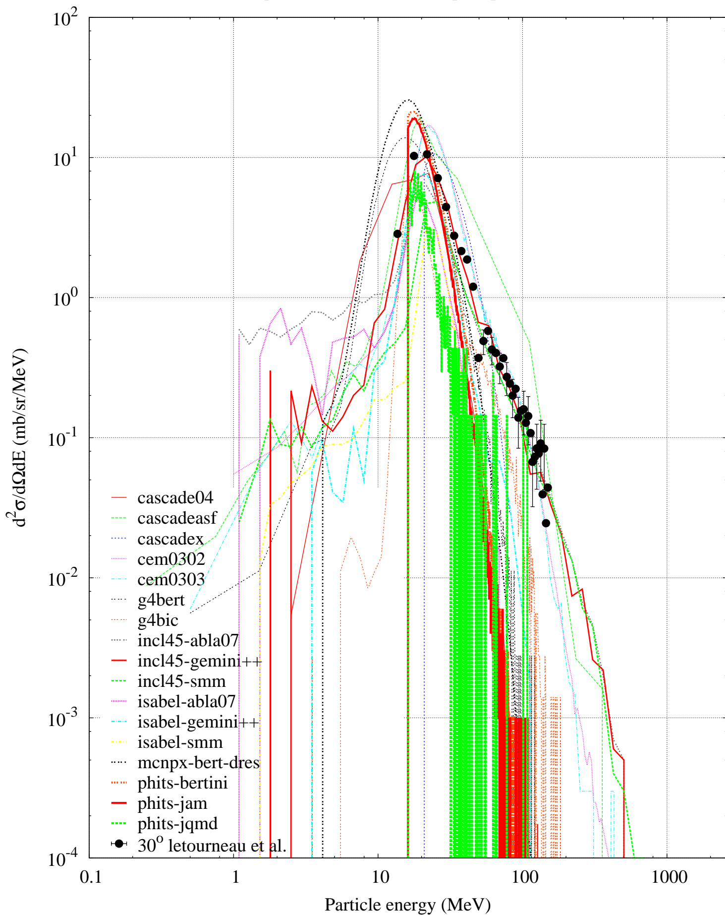
p (2500 MeV) + Au -- Alpha spectrum
