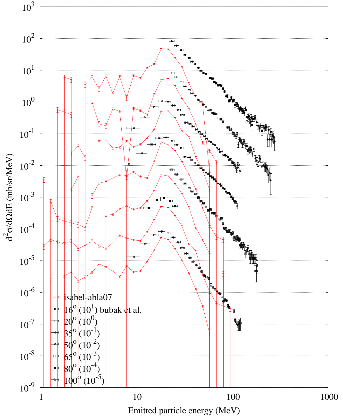
p (2500 MeV) + Au -- Helium-4 spectrum
