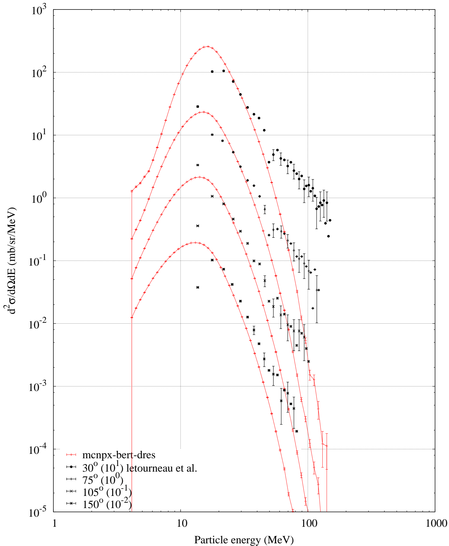
p (2500 MeV) + Au -- Alpha spectrum
