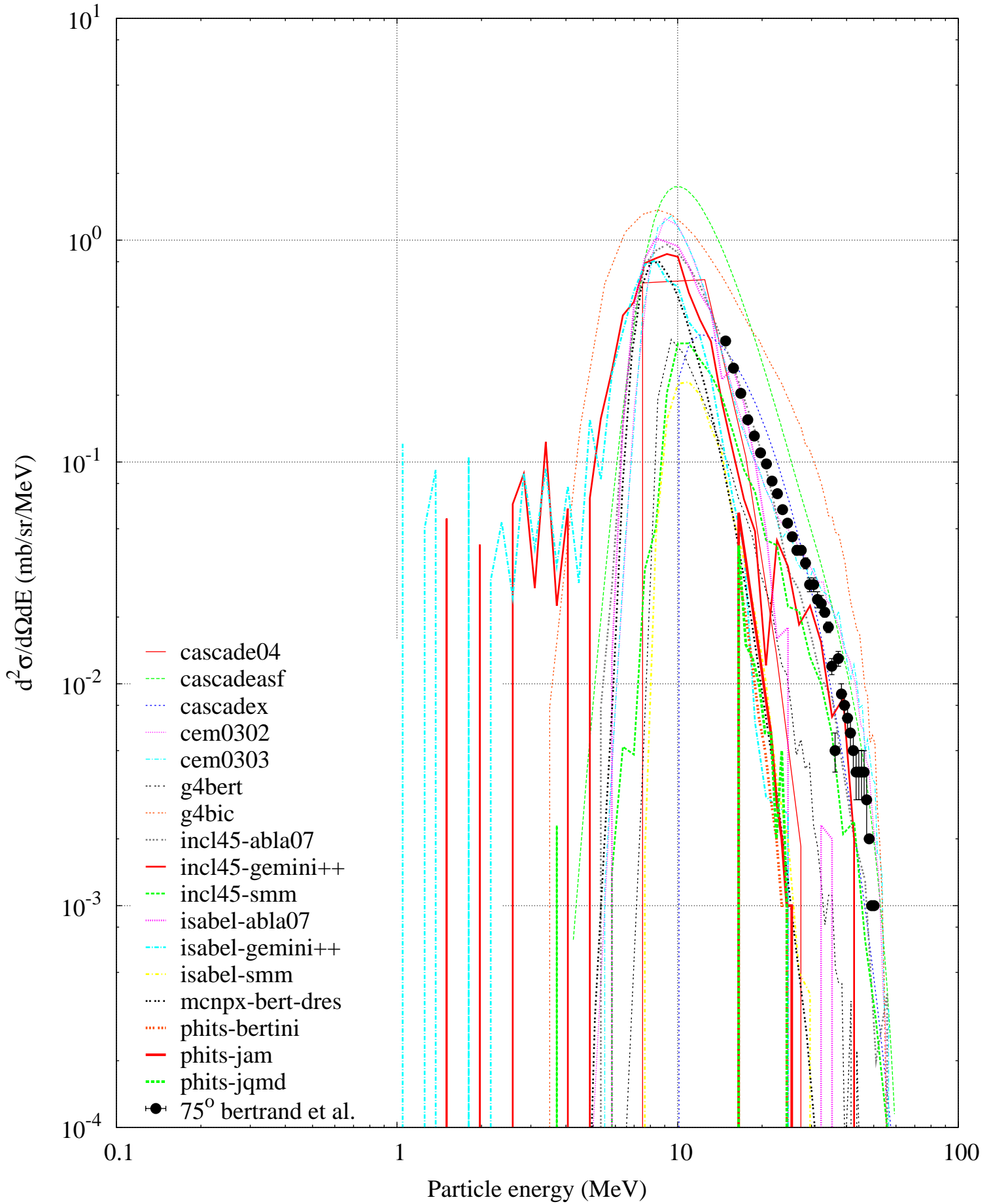
p (62 MeV) + Fe56 -- Alpha spectrum
