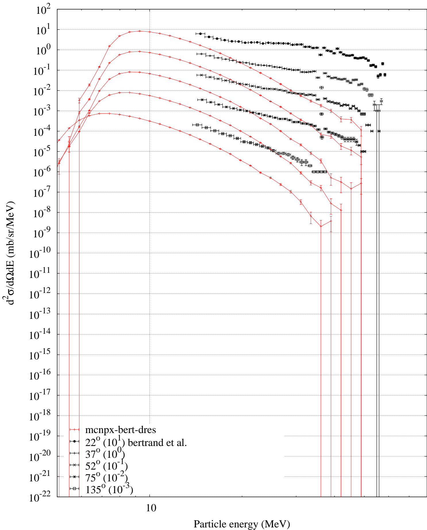
p (62 MeV) + Fe56 -- Alpha spectrum
