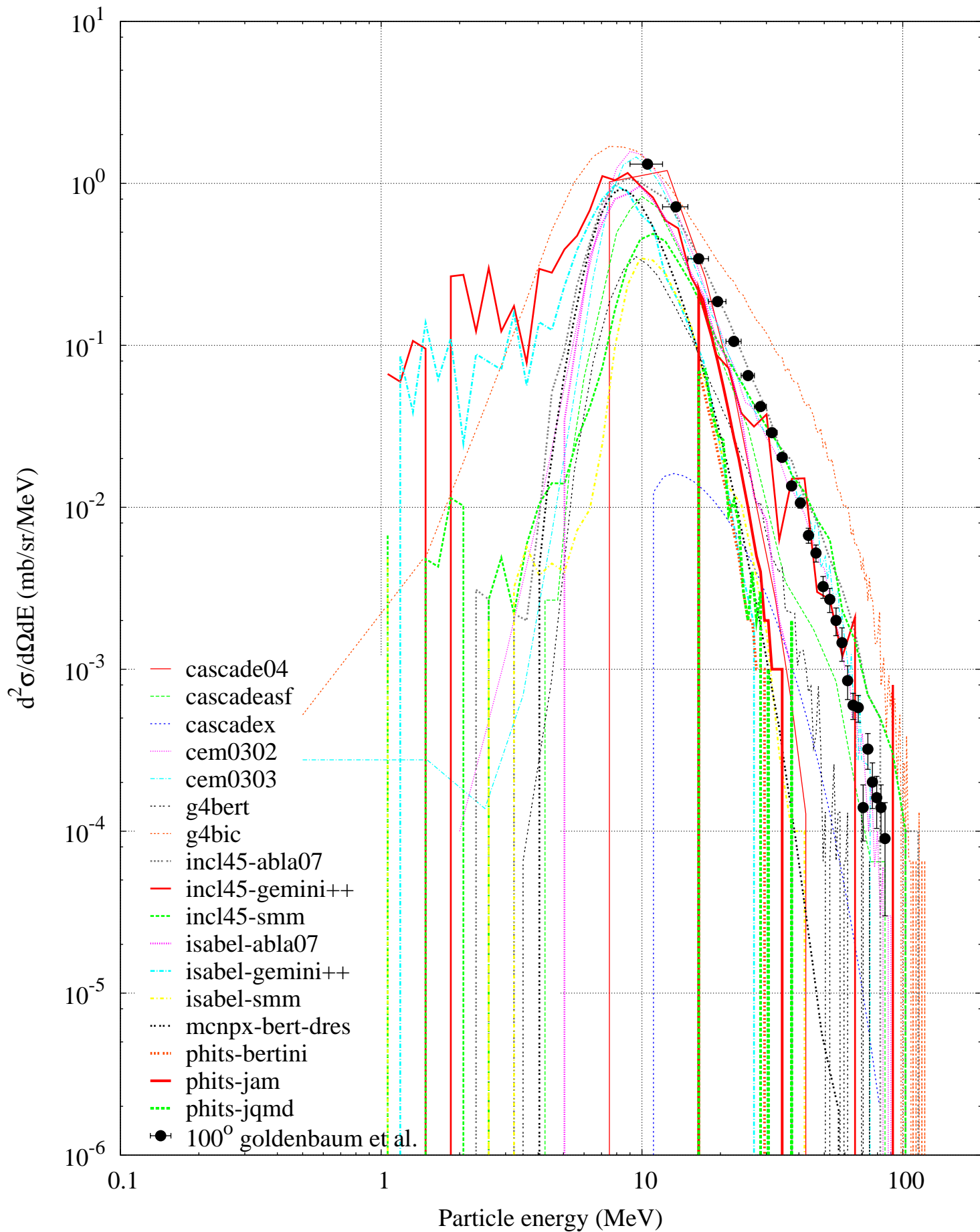
p (175 MeV) + Ni -- Alpha spectrum
