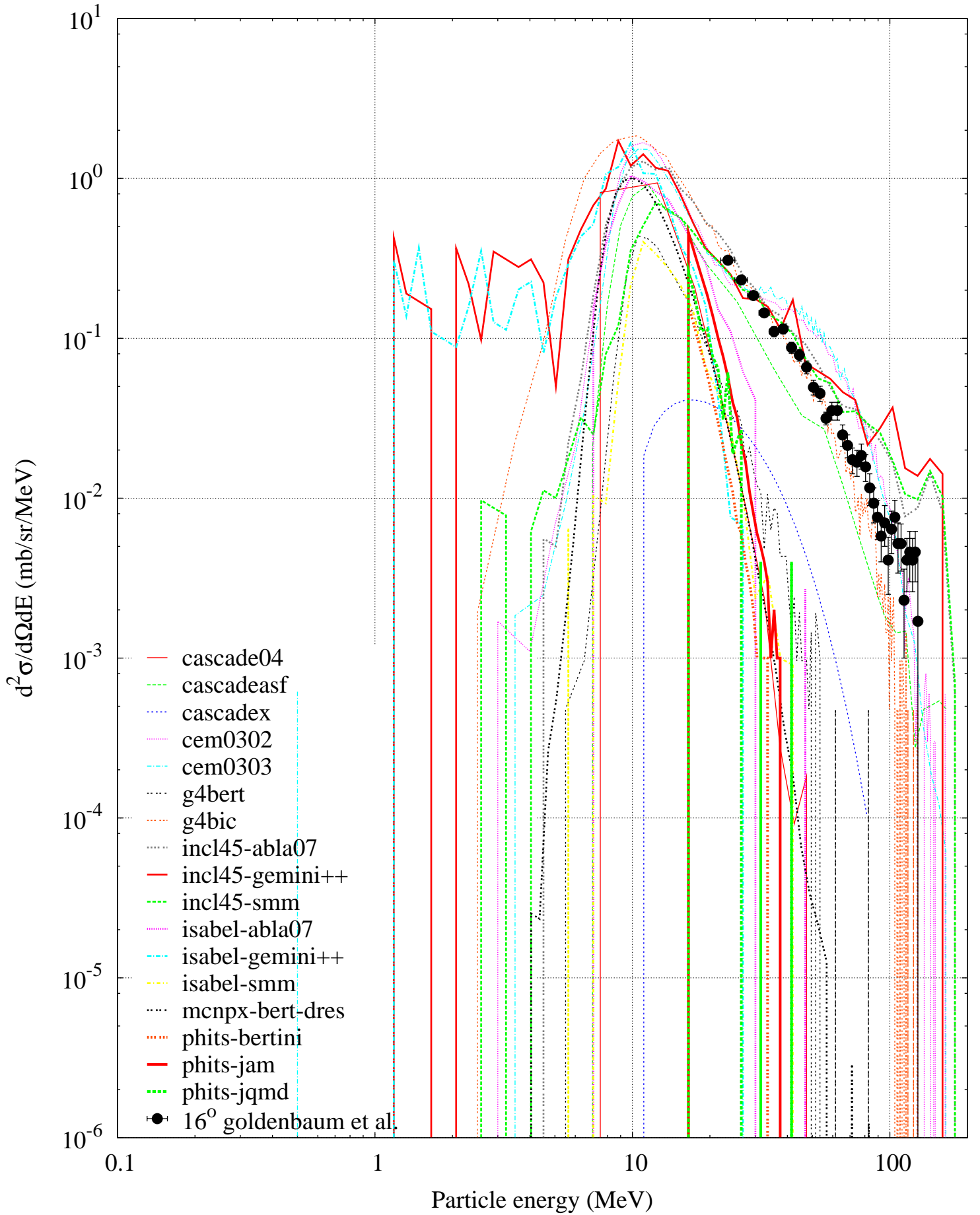
p (175 MeV) + Ni -- Alpha spectrum
