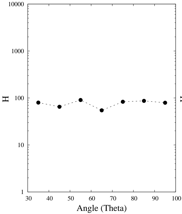
H factor - E_{\text{low}} (0-20 MeV)
