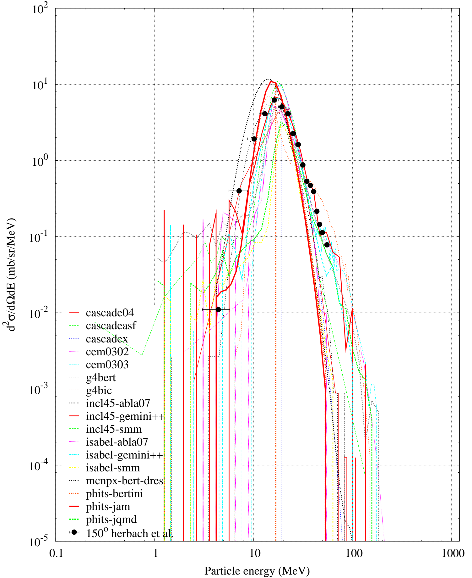
p (1200 MeV) + Ta -- Alpha spectrum
