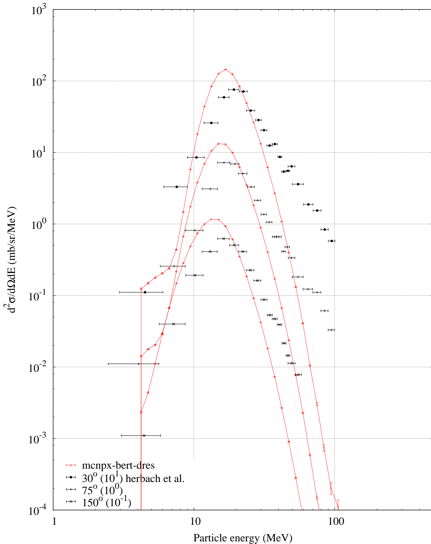
p (1200 MeV) + Ta -- Alpha spectrum
