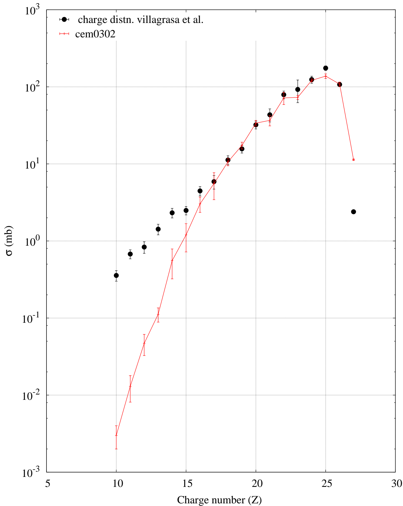
p (300 MeV) + Fe56 -- Residue charge production
