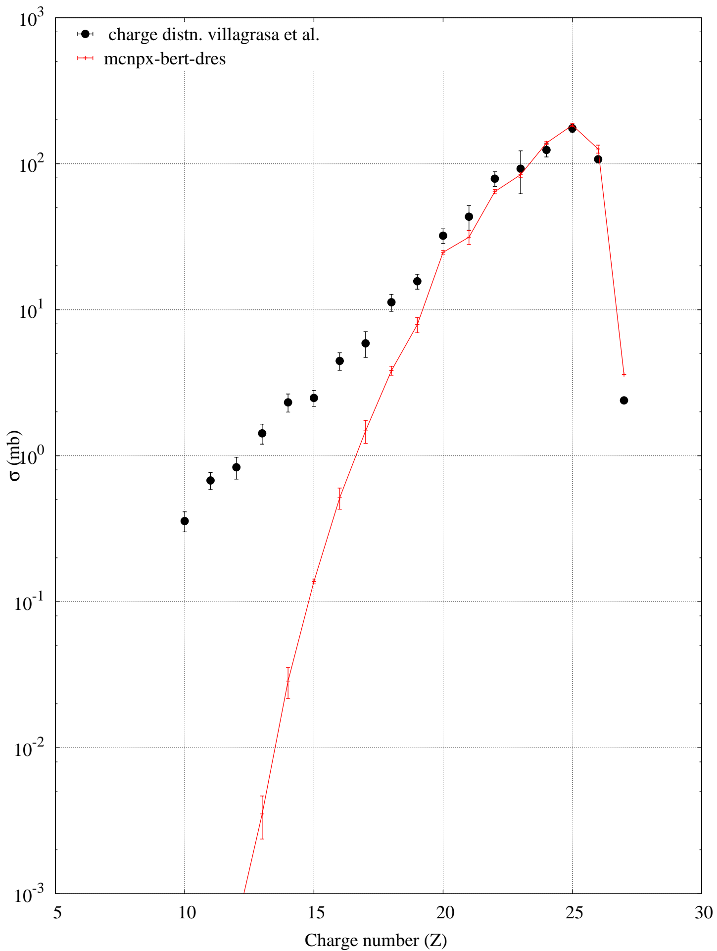
p (300 MeV) + Fe56 -- Residue charge production
