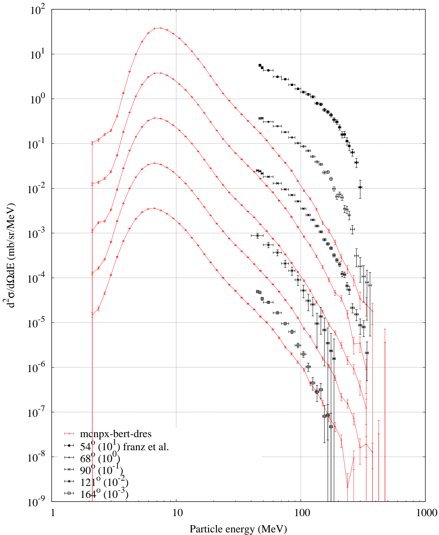
n (542 MeV) + Bi -- Deuteron spectrum
