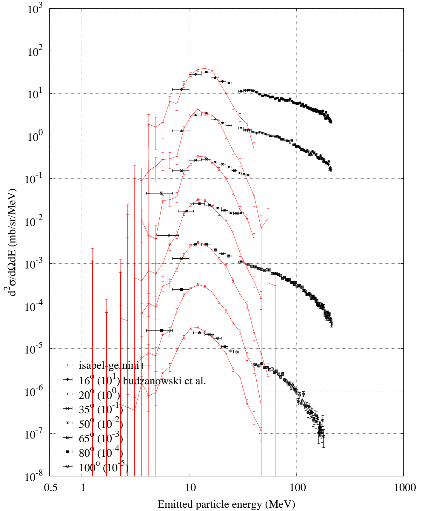
p (1200 MeV) + Au -- Deuteron spectrum
