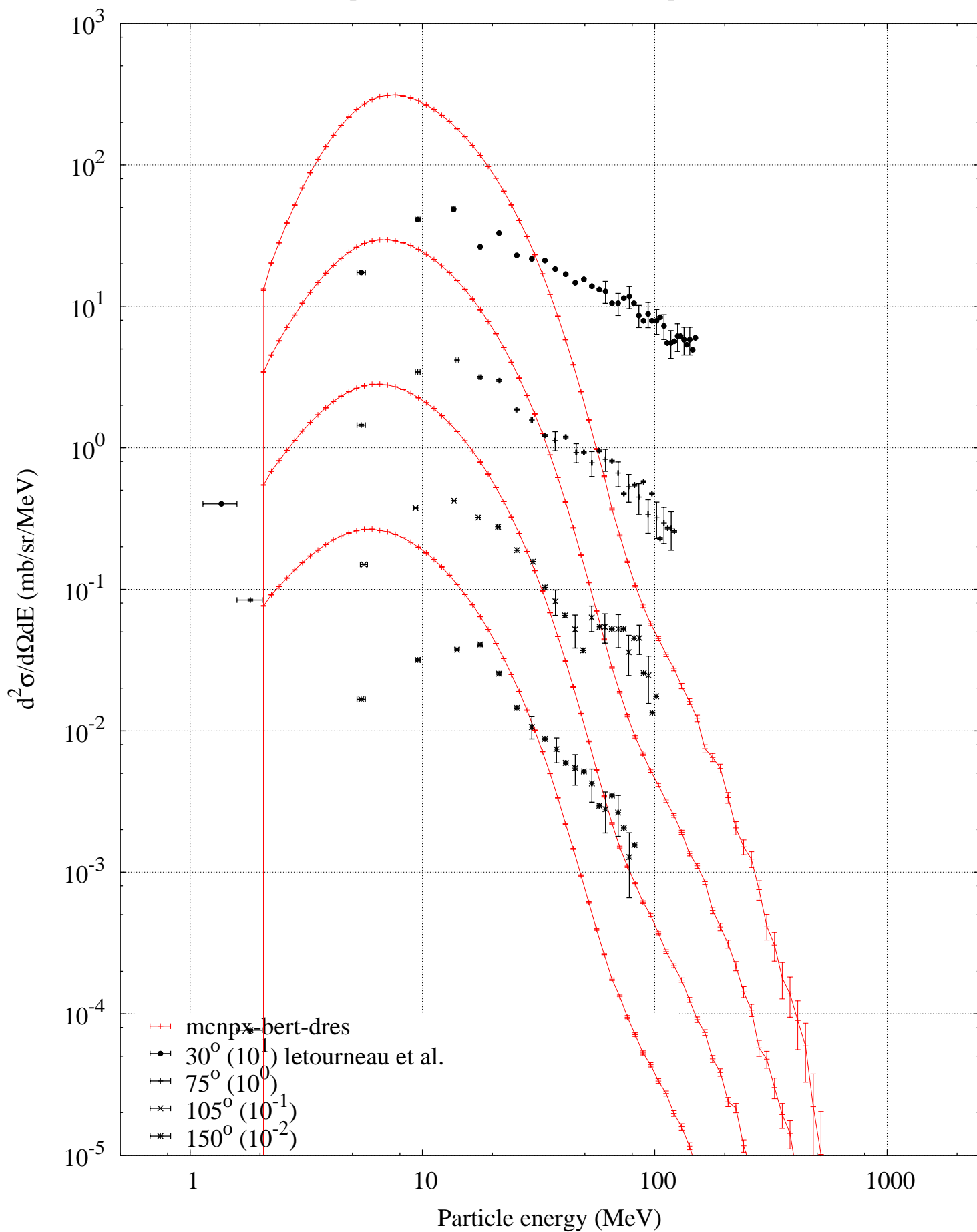
p (2500 MeV) + Au -- Deuteron spectrum
