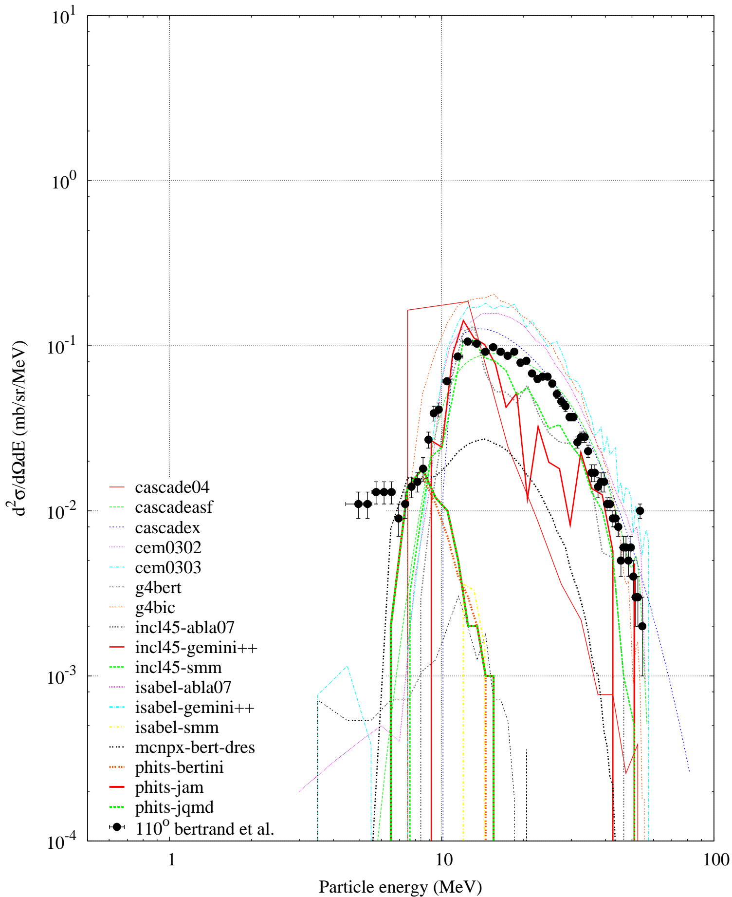
p (62 MeV) + Bi -- Deuteron spectrum
