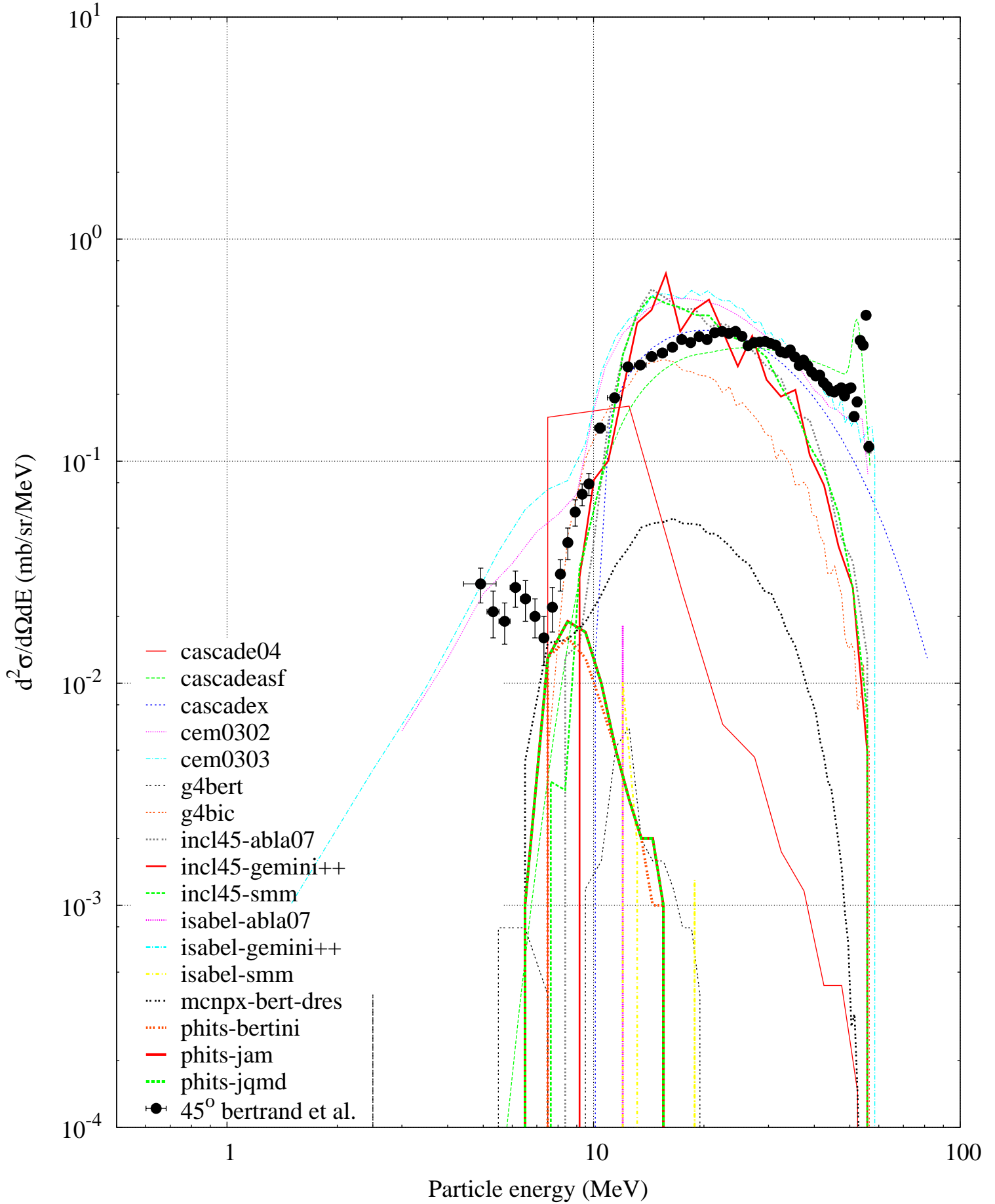
p (62 MeV) + Bi -- Deuteron spectrum
