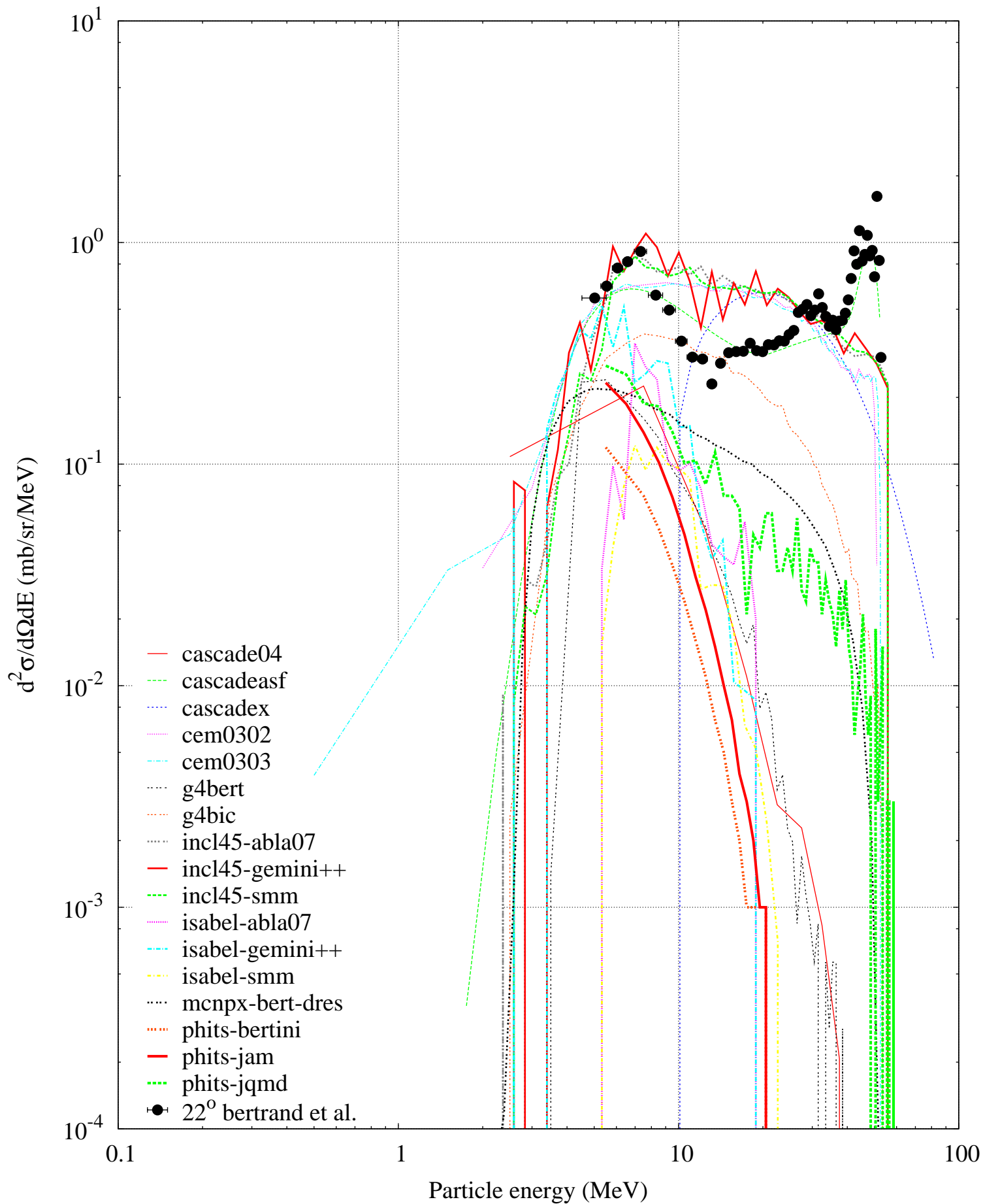
p (62 MeV) + Fe56 -- Deuteron spectrum
