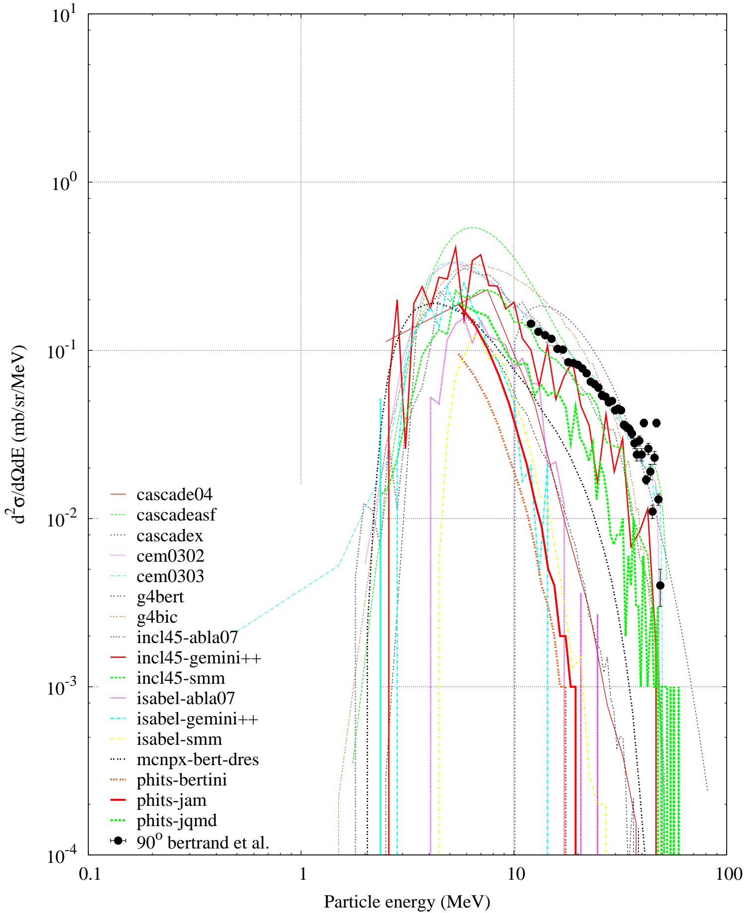
p (62 MeV) + Fe56 -- Deuteron spectrum
