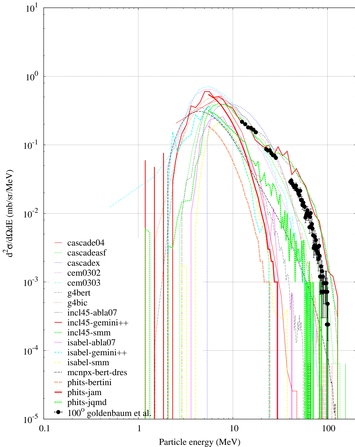
p (175 MeV) + Ni -- Deuteron spectrum
