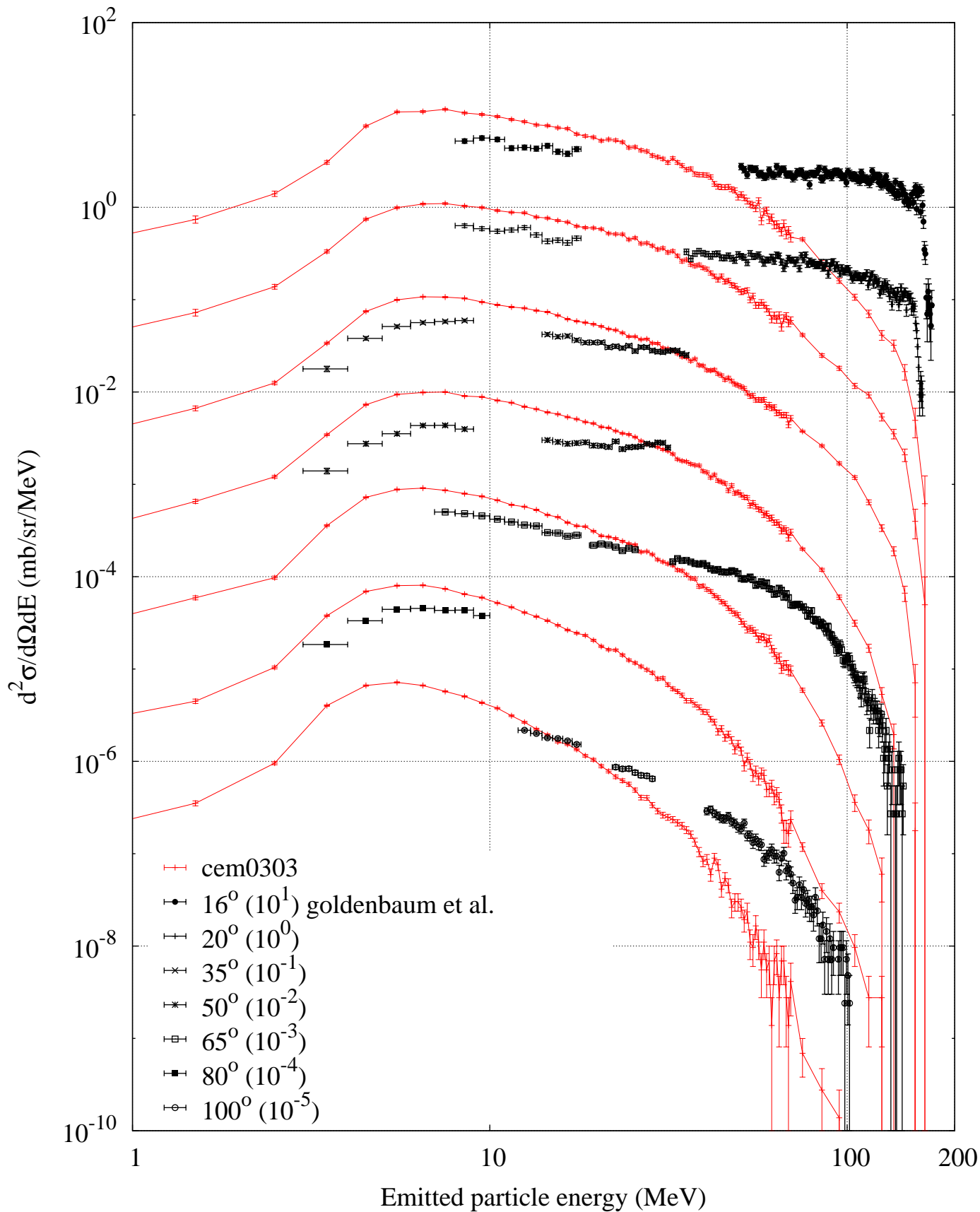
p (175 MeV) + Ni -- Deuteron spectrum
