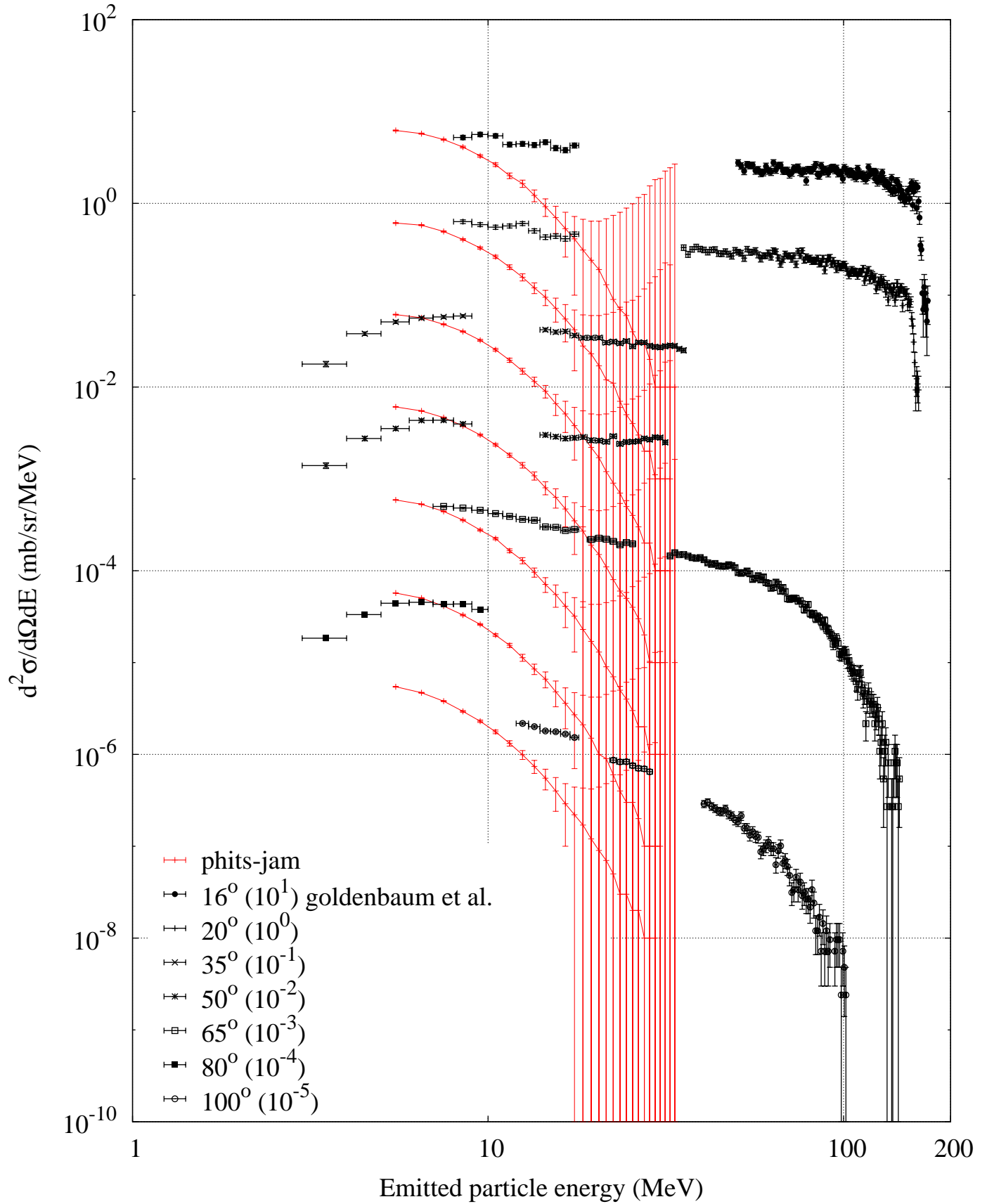
p (175 MeV) + Ni -- Deuteron spectrum
