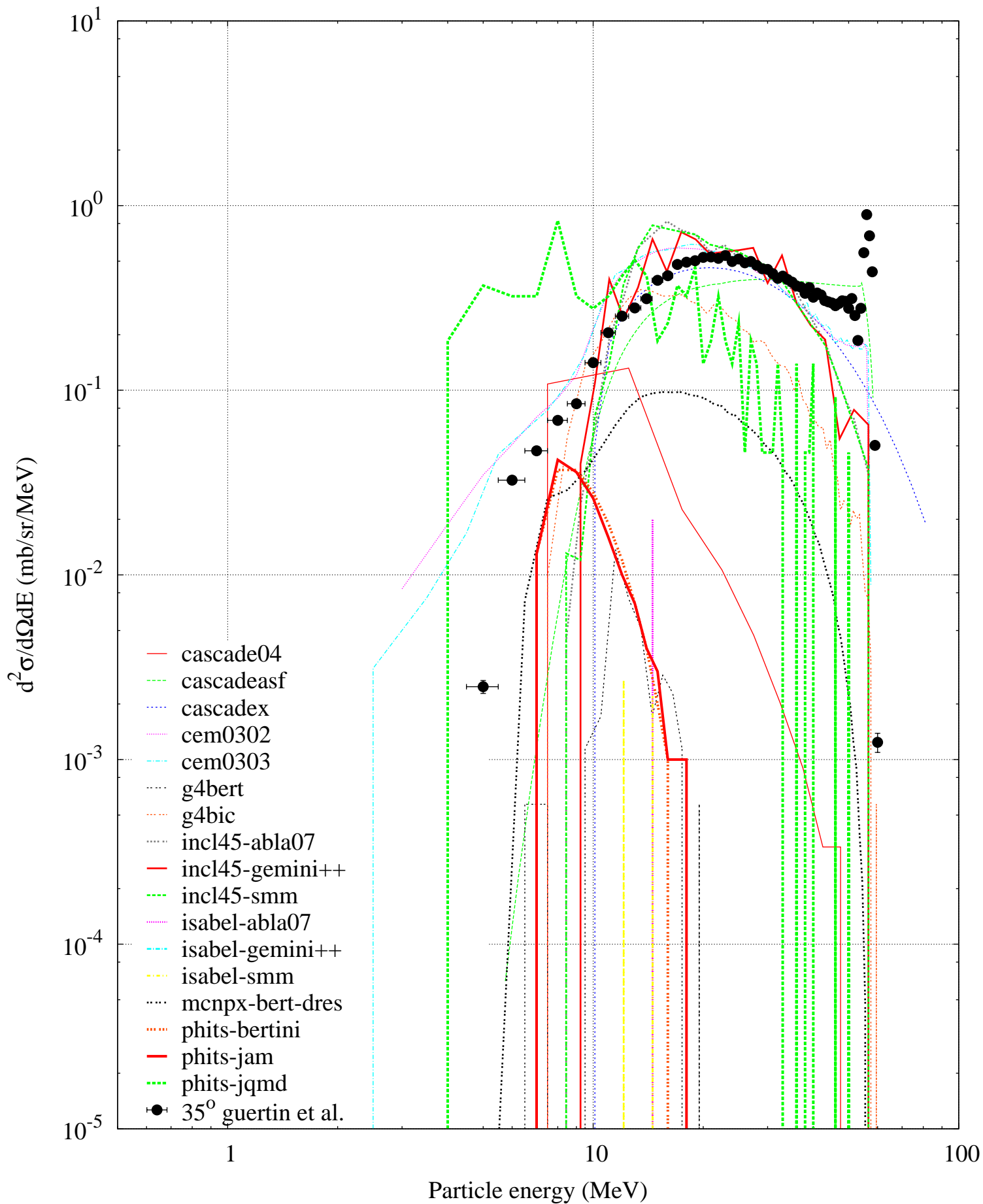
p (63 MeV) + Pb208 -- Deuteron spectrum
