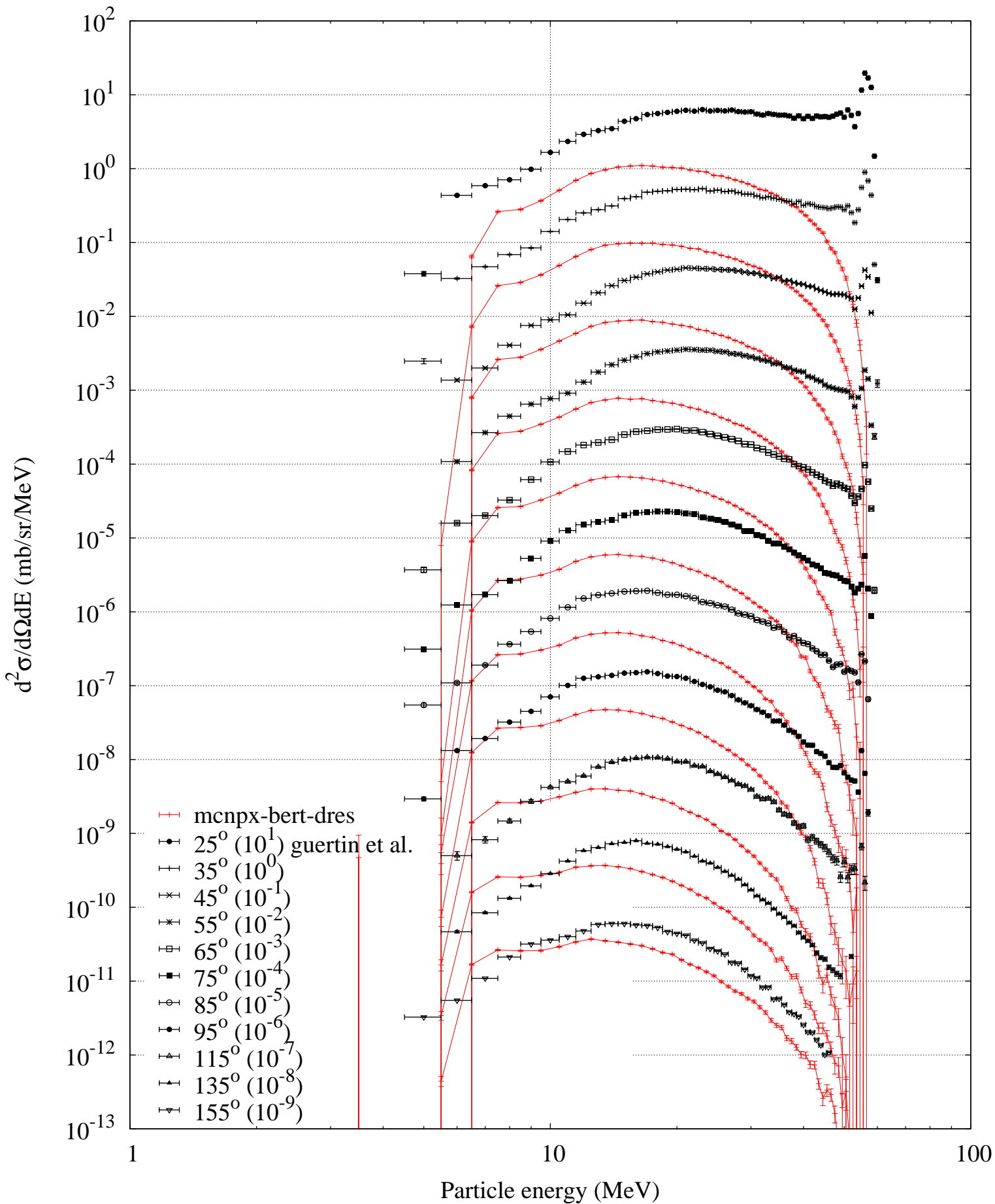
p (63 MeV) + Pb208 -- Deuteron spectrum
