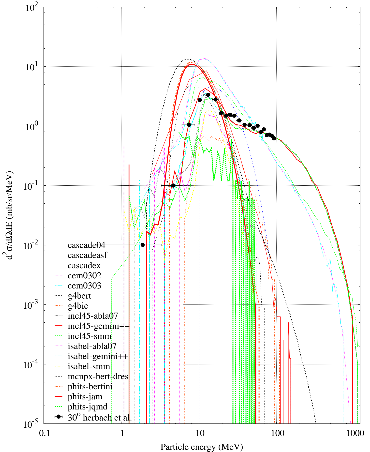
p (1200 MeV) + Ta -- Deuteron spectrum
