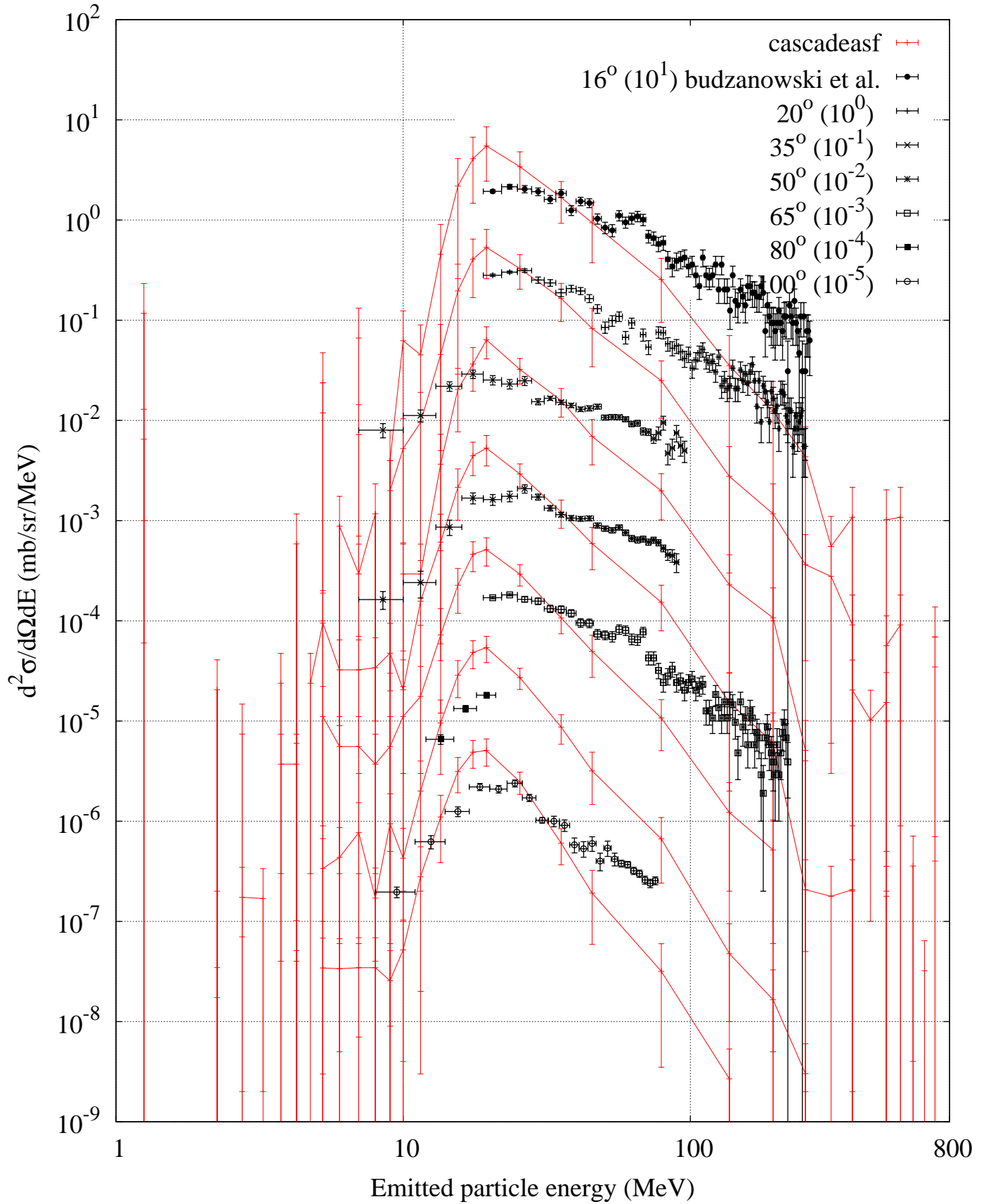
p (1200 MeV) + Au -- Helium-3 spectrum
