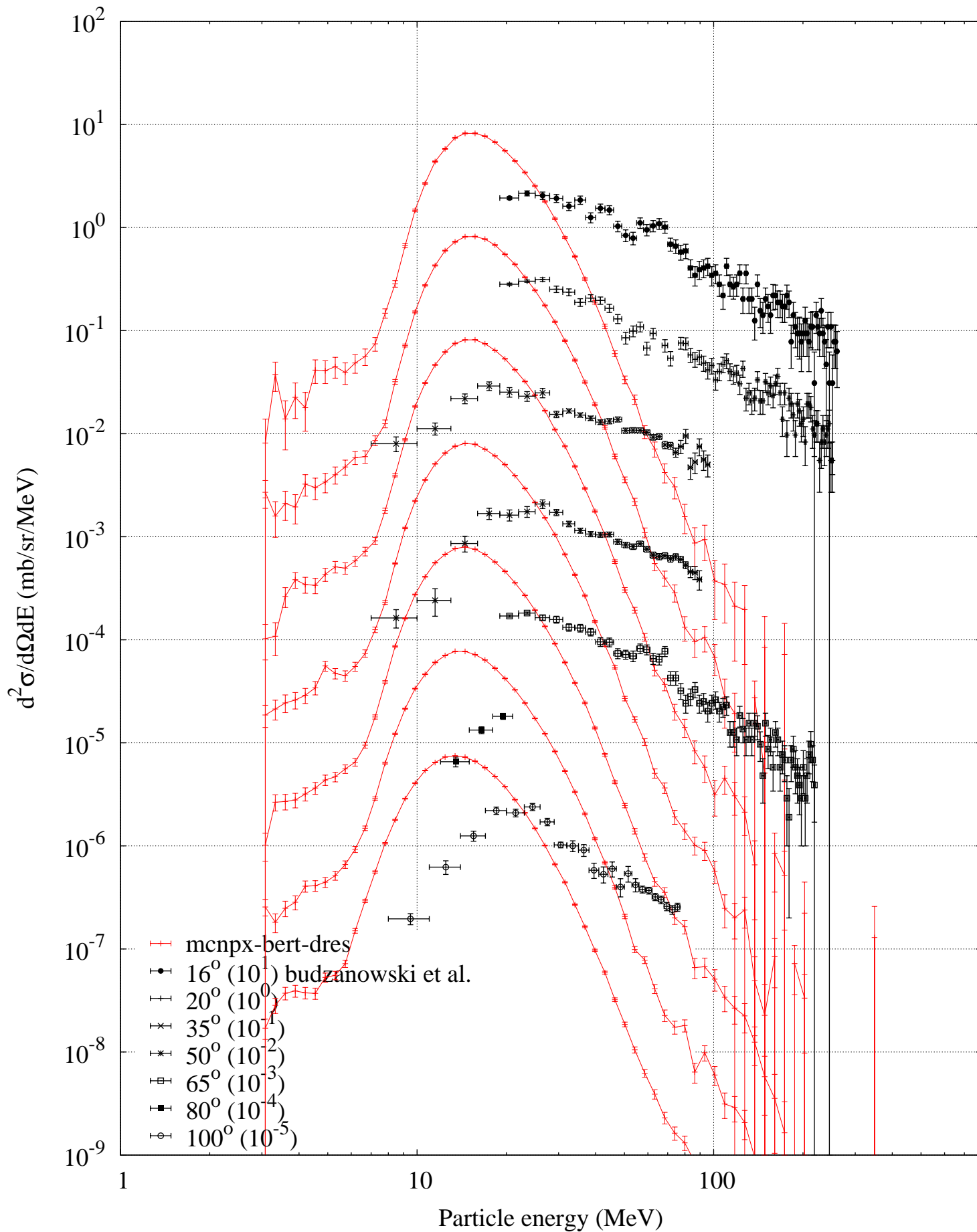
p (1200 MeV) + Au -- He3 spectrum
