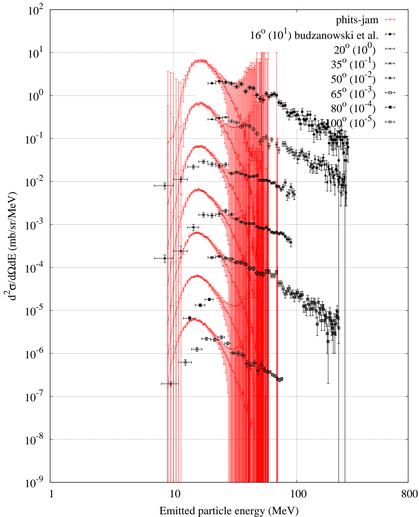
p (1200 MeV) + Au -- Helium-3 spectrum
