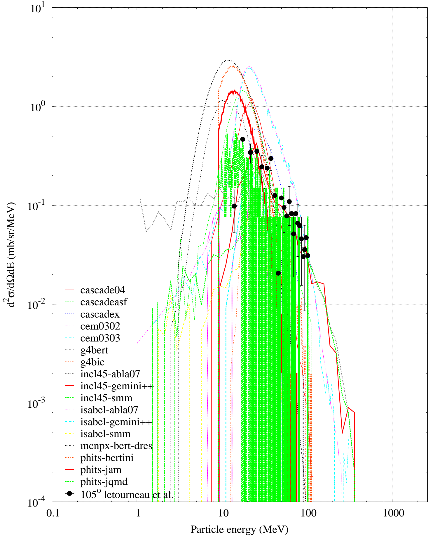
p (2500 MeV) + Au -- He3 spectrum
