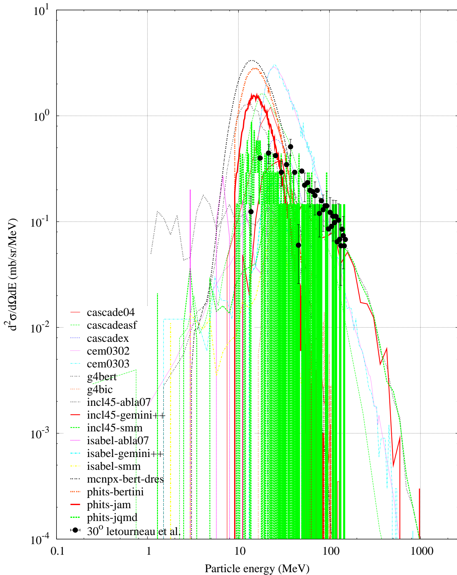
p (2500 MeV) + Au -- He3 spectrum
