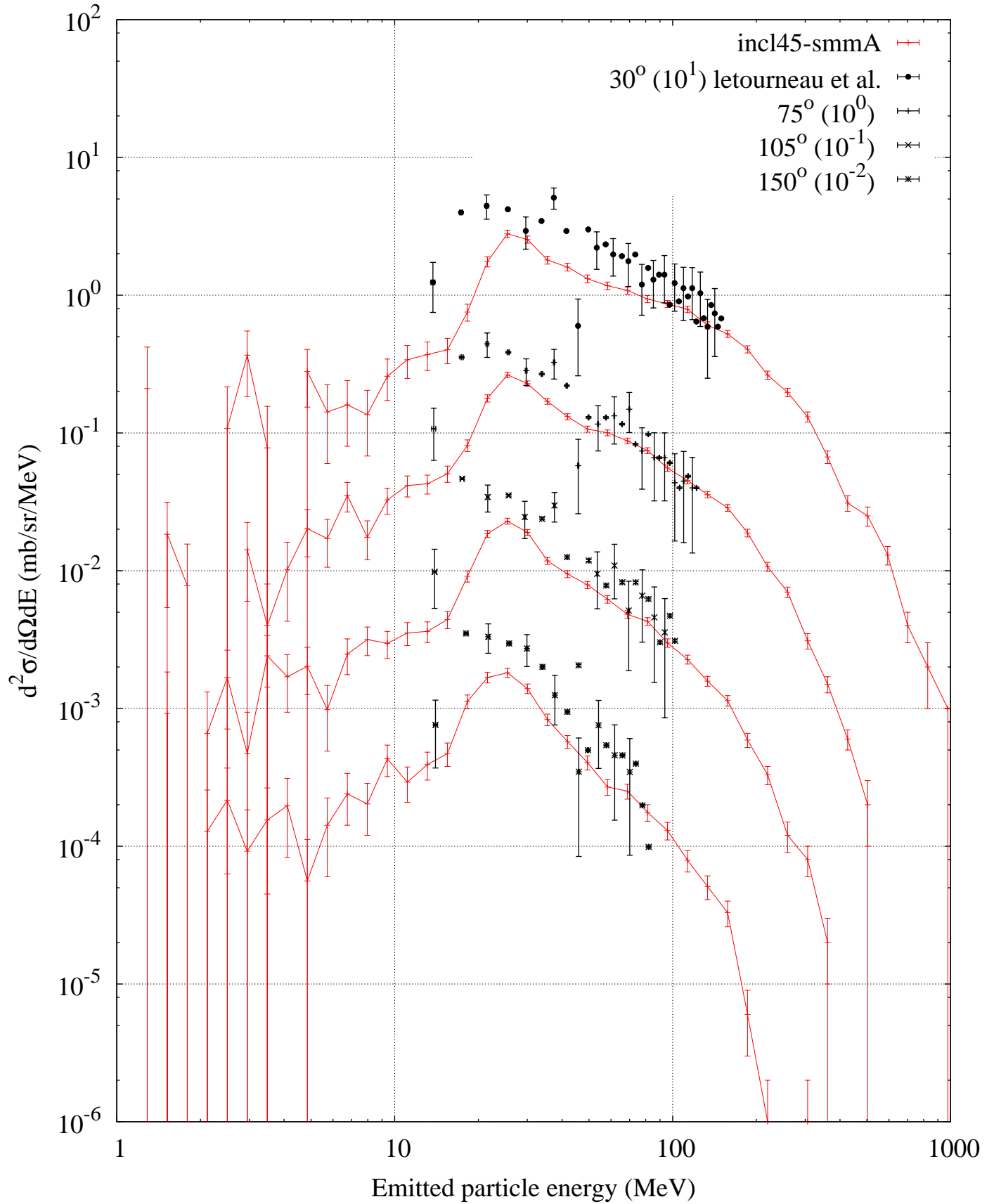
p (2500 MeV) + Au -- Helium-3 spectrum
