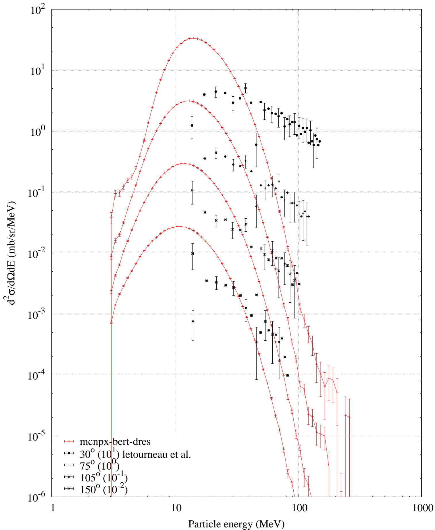
p (2500 MeV) + Au -- He3 spectrum
