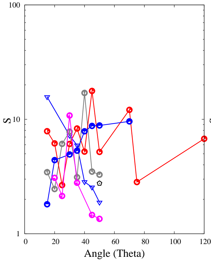
S factor - E_{\text{low}}(0-20 \text{ MeV})
