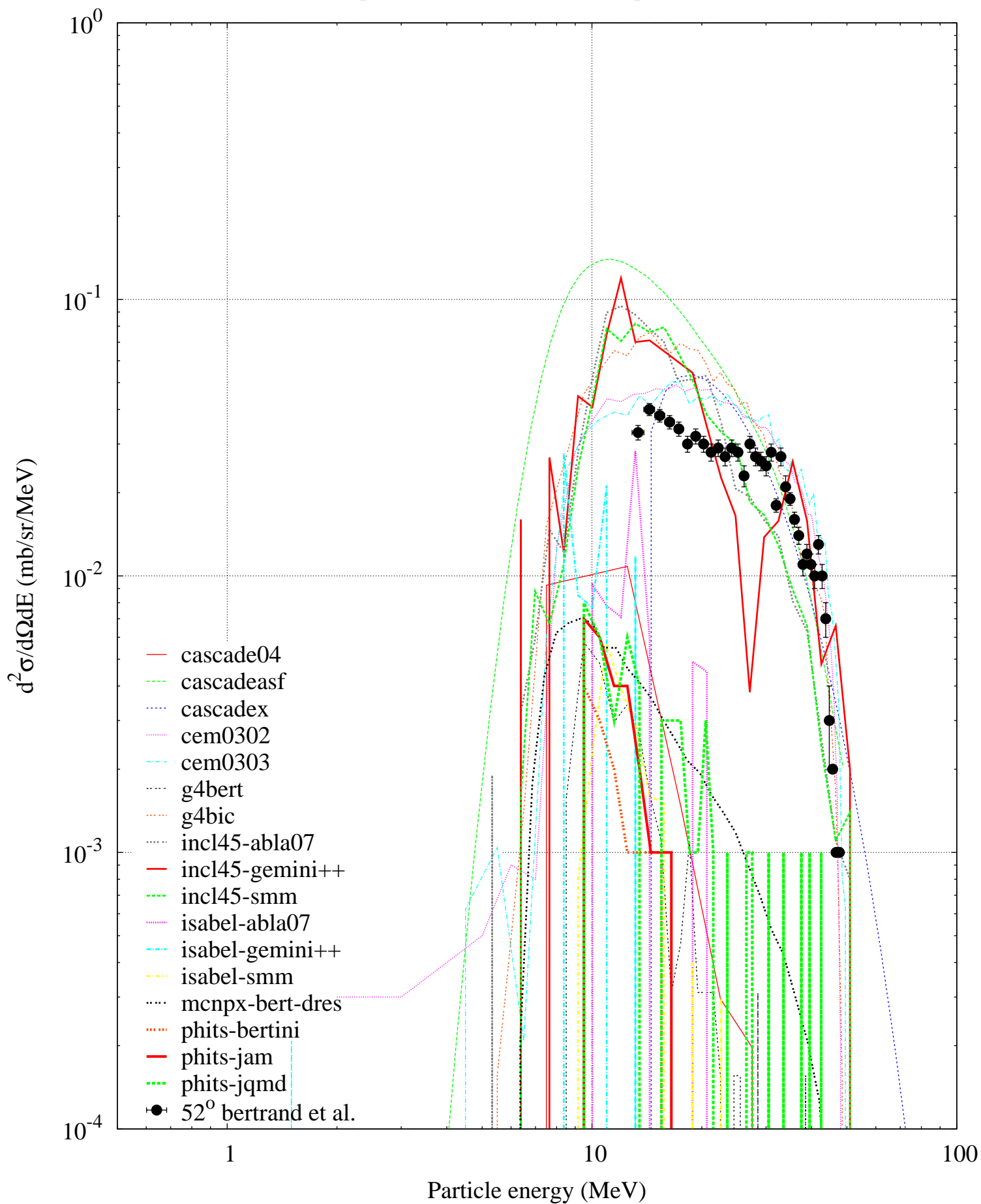
p (62 MeV) + Fe56 -- He3 spectrum
