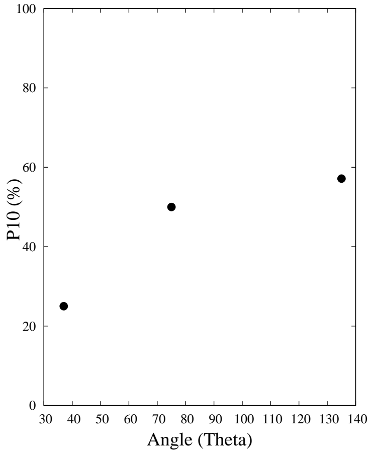
P10 factor - E_{\text{low}} (0-20 MeV)
