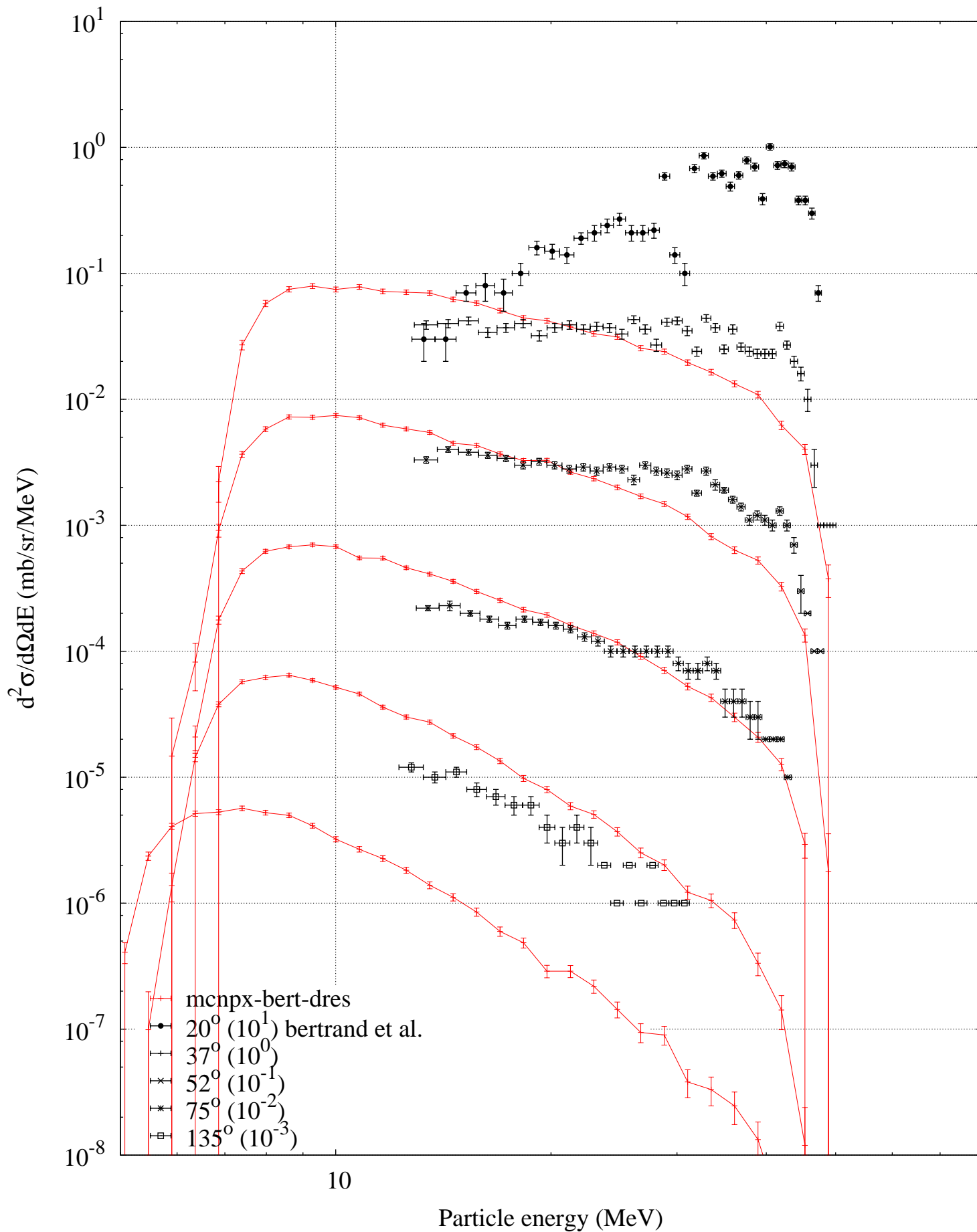
p (62 MeV) + Fe56 -- He3 spectrum
