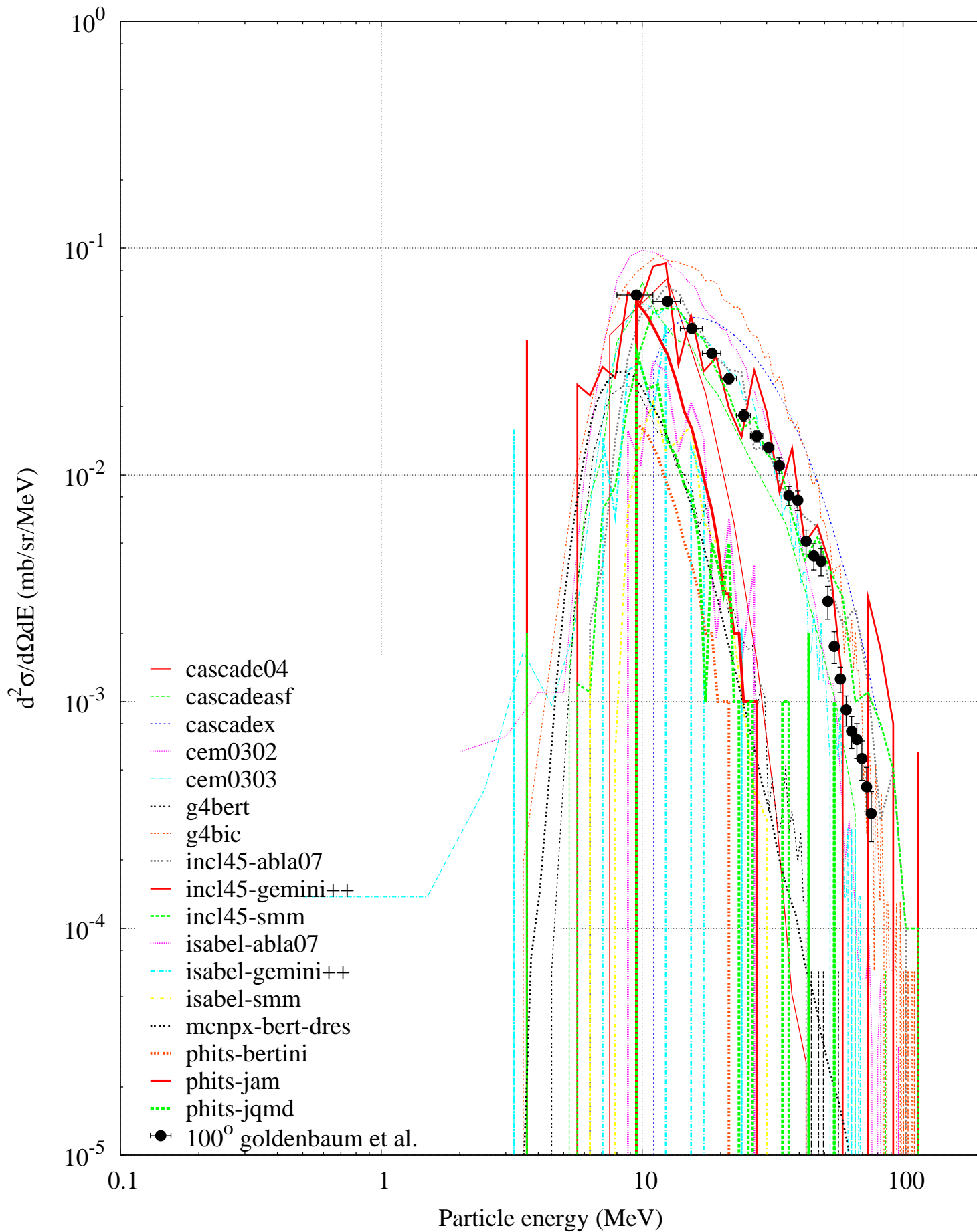
p (175 MeV) + Ni -- He3 spectrum
