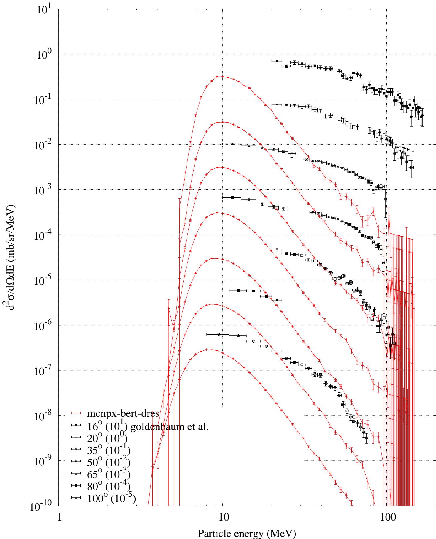
p (175 MeV) + Ni -- He3 spectrum
