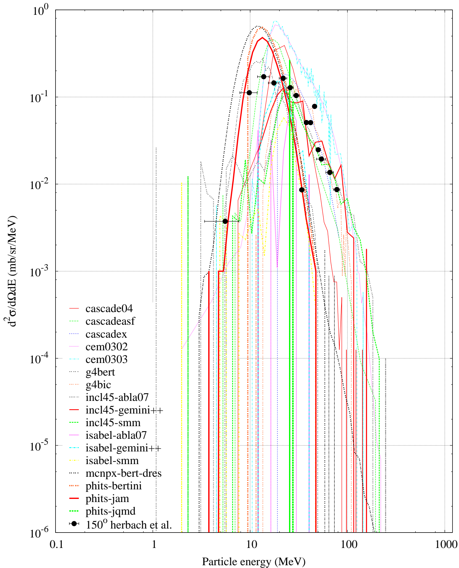
p (1200 MeV) + Ta -- He3 spectrum
