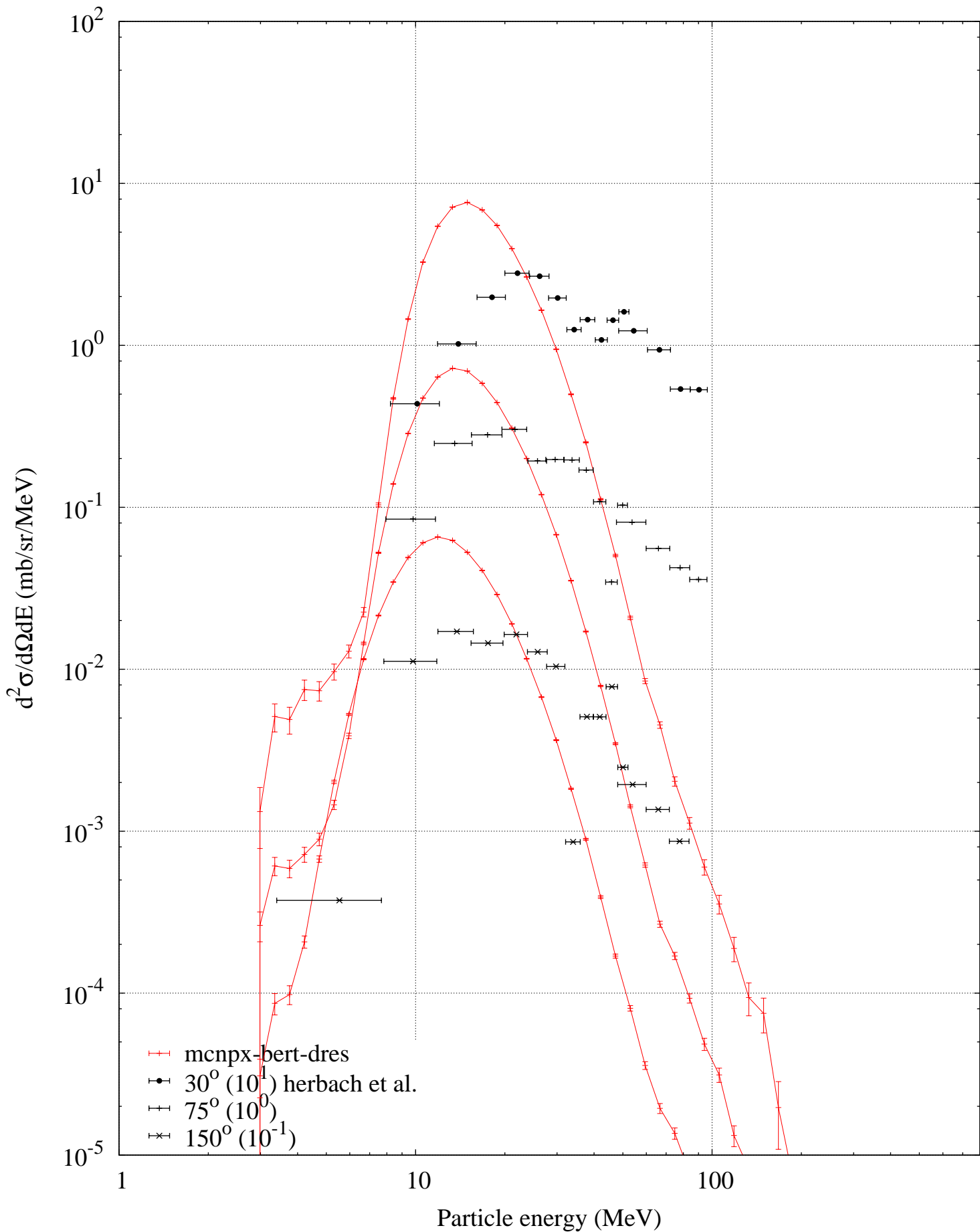
p (1200 MeV) + Ta -- He3 spectrum
