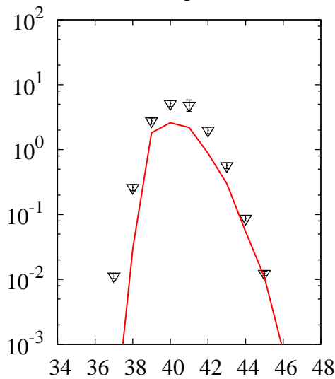
^{56}\text{Fe}(p,x)\text{K}
