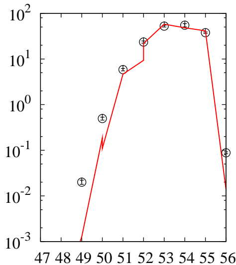
^{56}\text{Fe}(p,x)\text{Mn}
