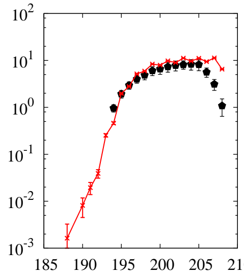
^{208}\text{Pb}(p,x)\text{Bi}
