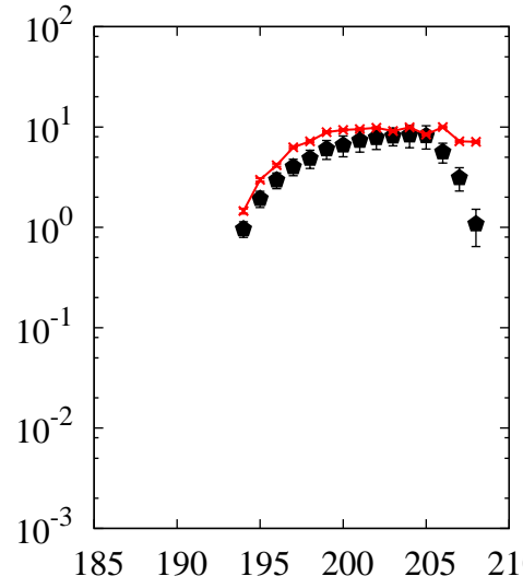
^{208}\text{Pb}(p,x)\text{Bi}
