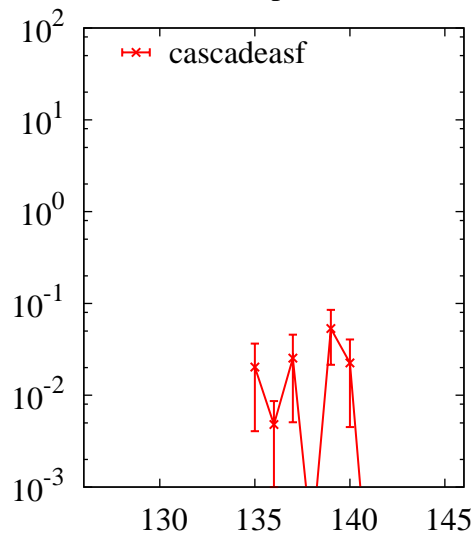
^{208}\text{Pb}(p,x)\text{Pr}
