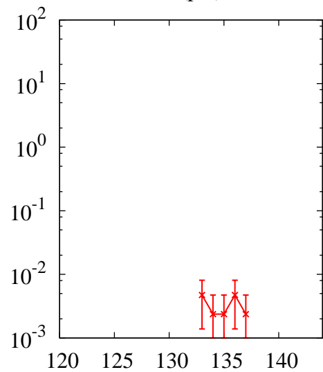
^{208}\text{Pb}(p,x)\text{La}
