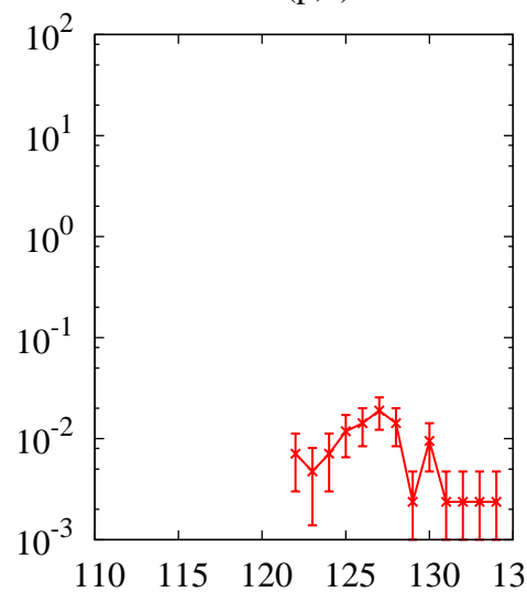
^{208}\text{Pb}(p,x)\text{Xe}
