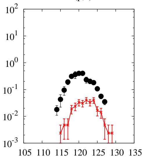
^{208}\text{Pb}(p,x)\text{Te}
