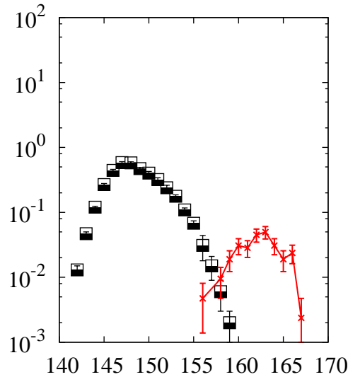
^{208}\text{Pb}(p,x)\text{Tb}
