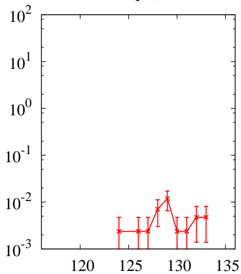
^{208}\text{Pb}(p,x)\text{Cs}
