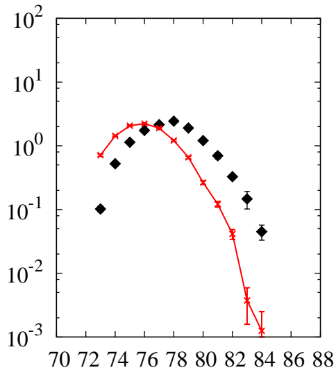
^{208}\text{Pb}(p,x)\text{Se}
