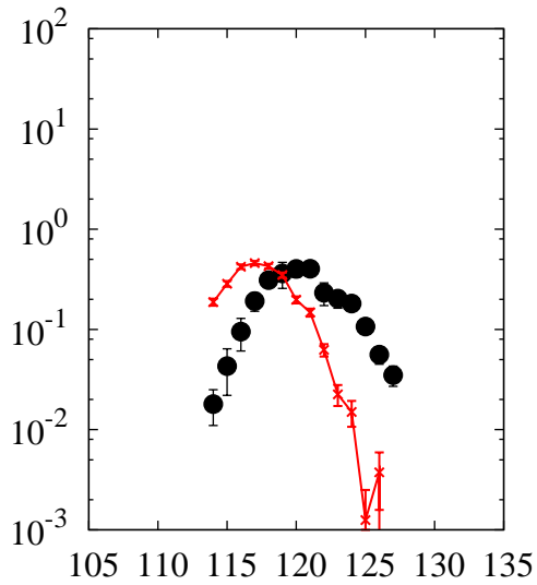
^{208}\text{Pb}(p,x)\text{Te}
