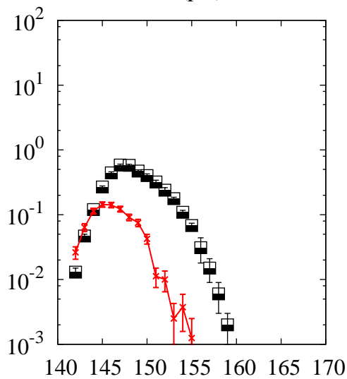
^{208}\text{Pb}(p,x)\text{Tb}
