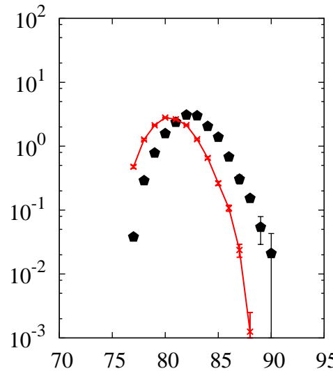
^{208}\text{Pb}(p,x)\text{Kr}
