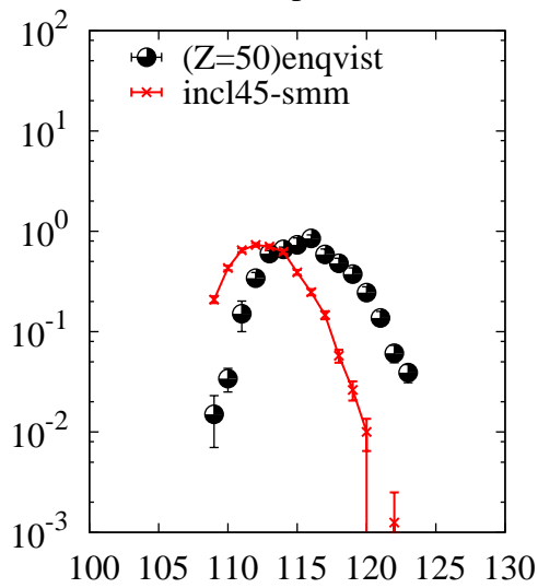
^{208}\text{Pb}(p,x)\text{Sn}
