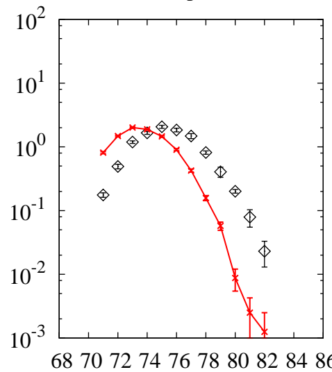
^{208}\text{Pb}(p,x)\text{As}
