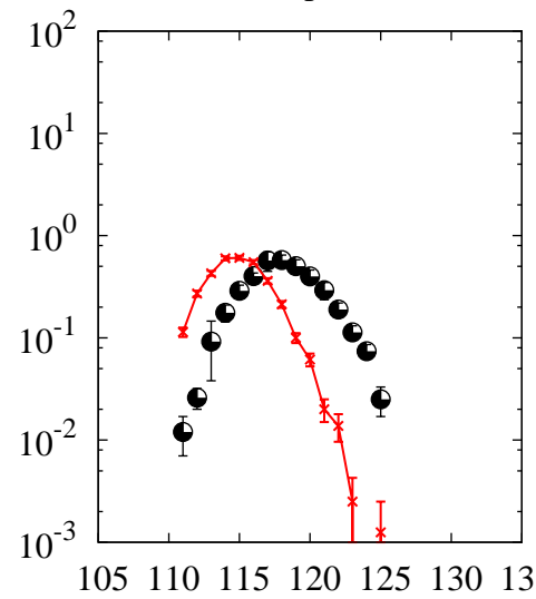
^{208}\text{Pb}(p,x)\text{Sb}
