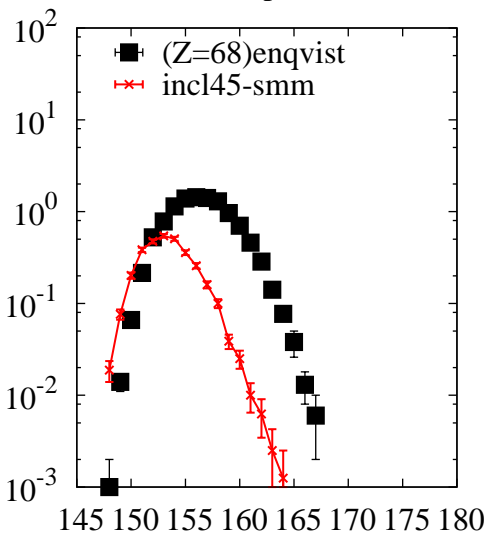
^{208}\text{Pb}(p,x)\text{Er}
