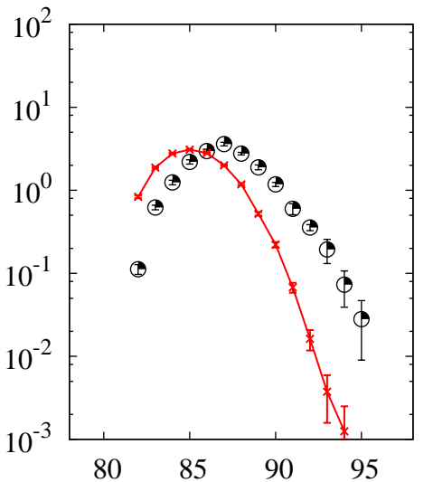
^{208}\text{Pb}(p,x)\text{Sr}
