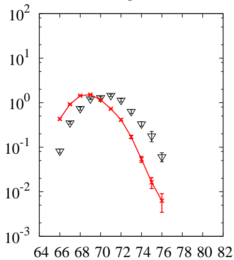
^{208}\text{Pb}(p,x)\text{Ga}
