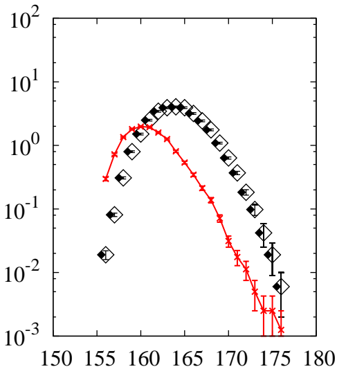
^{208}\text{Pb}(p,x)\text{Lu}
