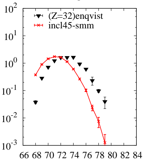
^{208}\text{Pb}(p,x)\text{Ge}
