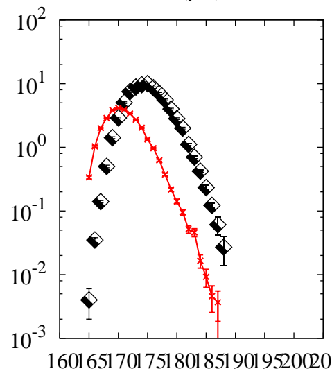
^{208}\text{Pb}(p,x)\text{Re}
