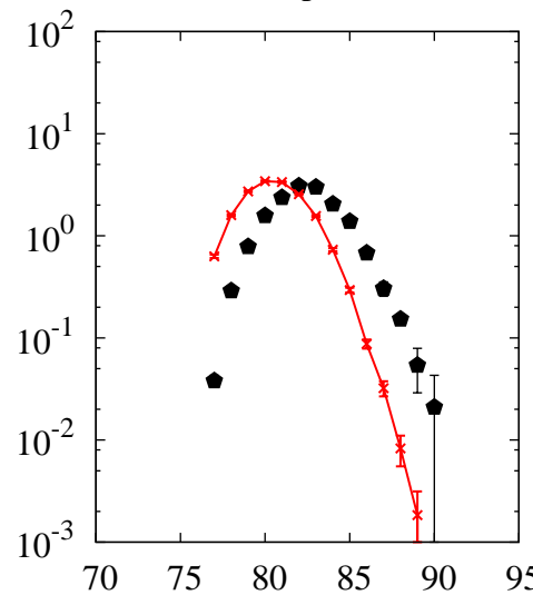
^{208}\text{Pb}(p,x)\text{Kr}
