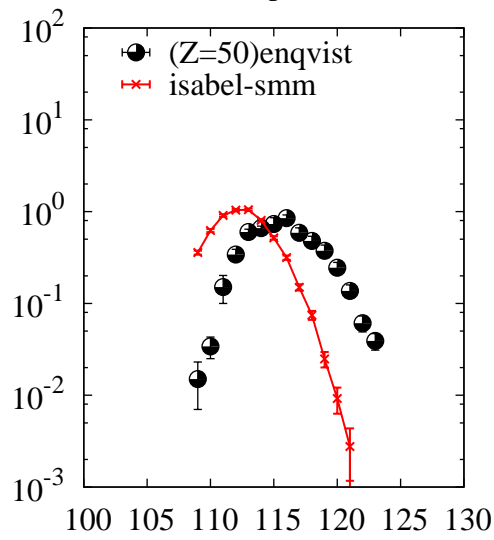
^{208}\text{Pb}(p,x)\text{Sn}
