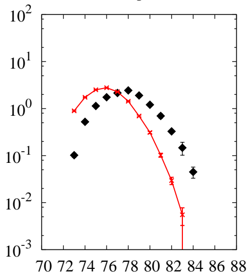
^{208}\text{Pb}(p,x)\text{Se}
