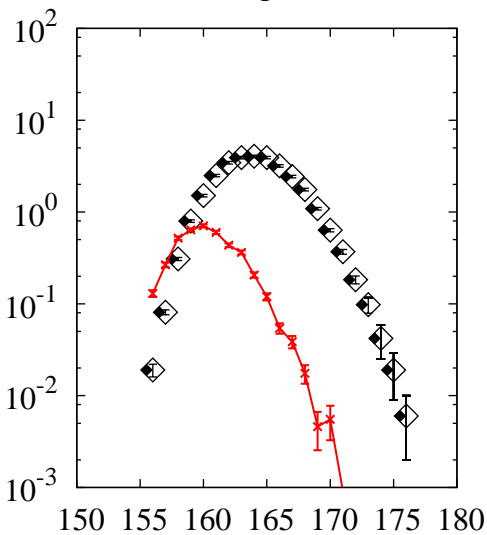
^{208}\text{Pb}(p,x)\text{Lu}
