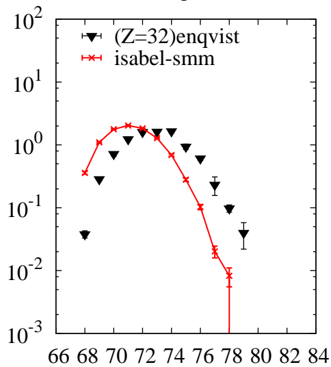
^{208}\text{Pb}(p,x)\text{Ge}
