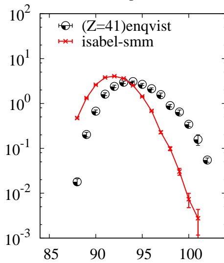
^{208}\text{Pb}(p,x)\text{Nb}
