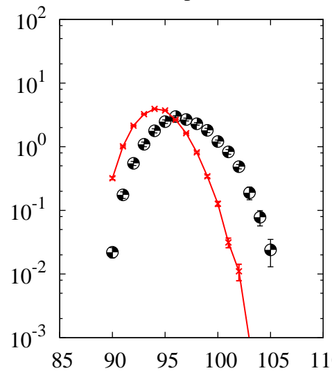
^{208}\text{Pb}(p,x)\text{Mo}
