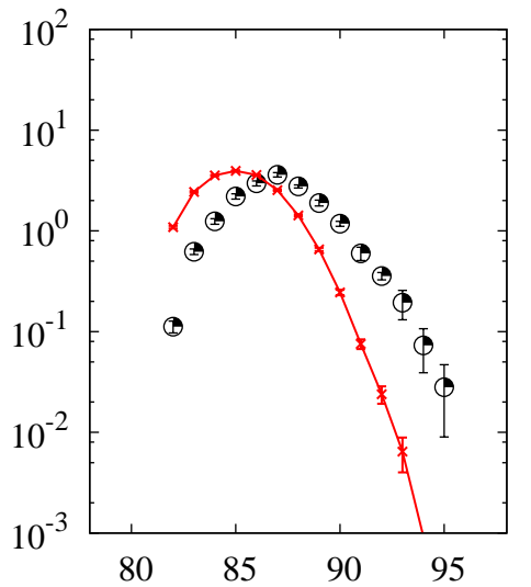
^{208}\text{Pb}(p,x)\text{Sr}
