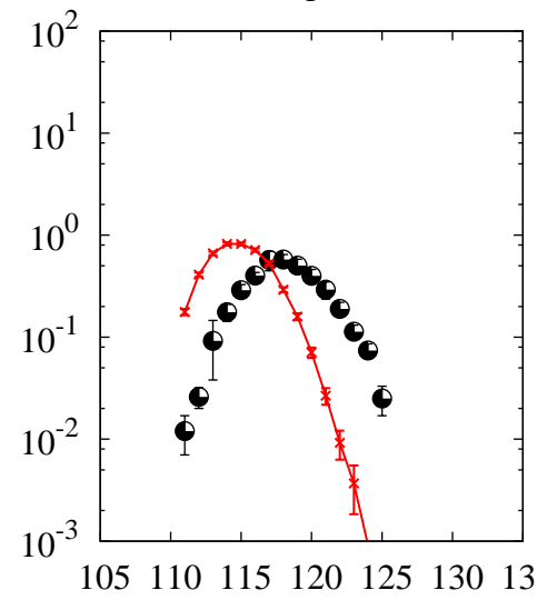
^{208}\text{Pb}(p,x)\text{Sb}
