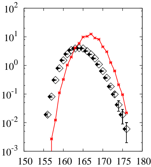
^{208}\text{Pb}(p,x)\text{Lu}
