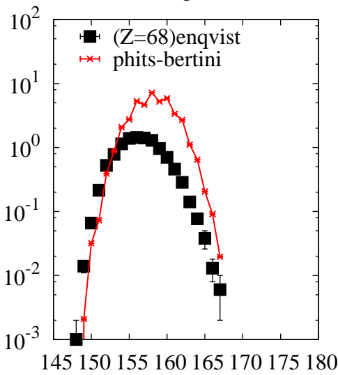
^{208}\text{Pb}(p,x)\text{Er}
